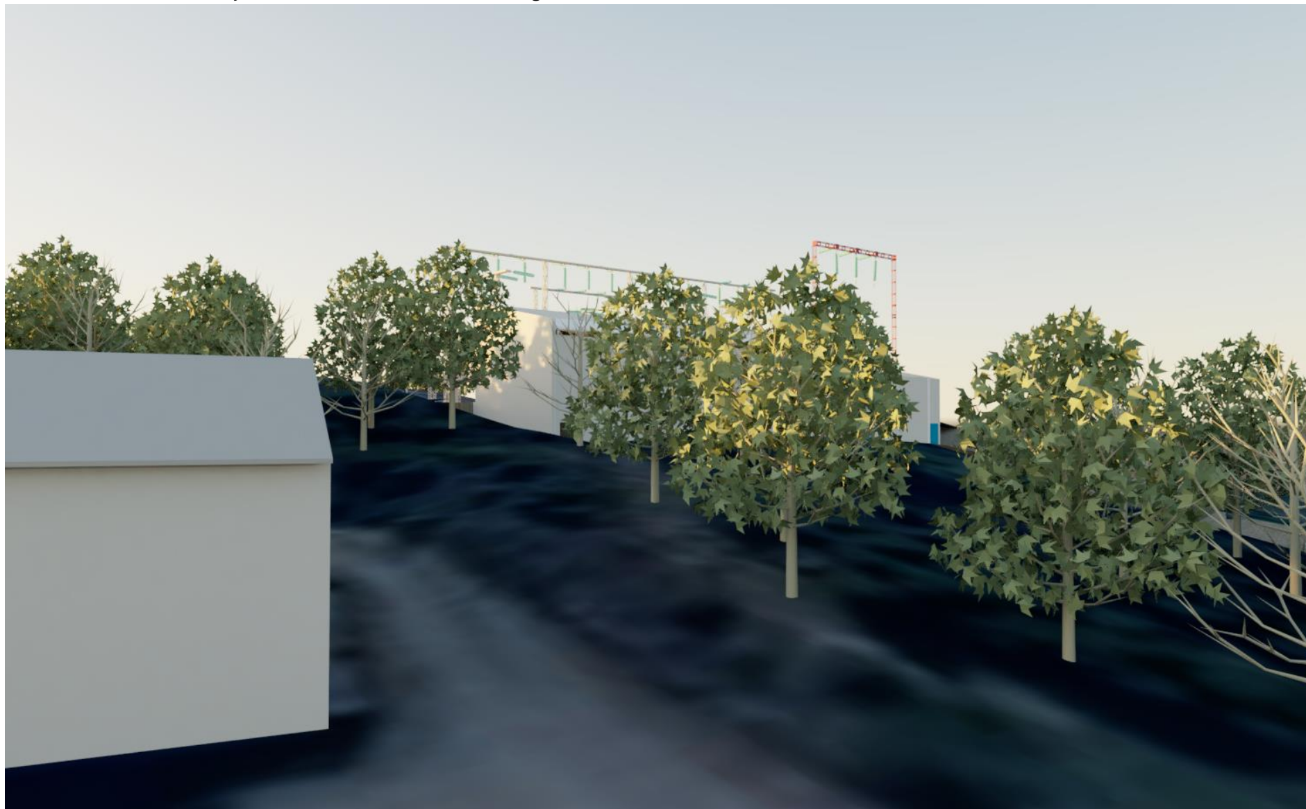
Sørtveit transformatorstasjon sett fra nærmeste nabo, retning sørvest
