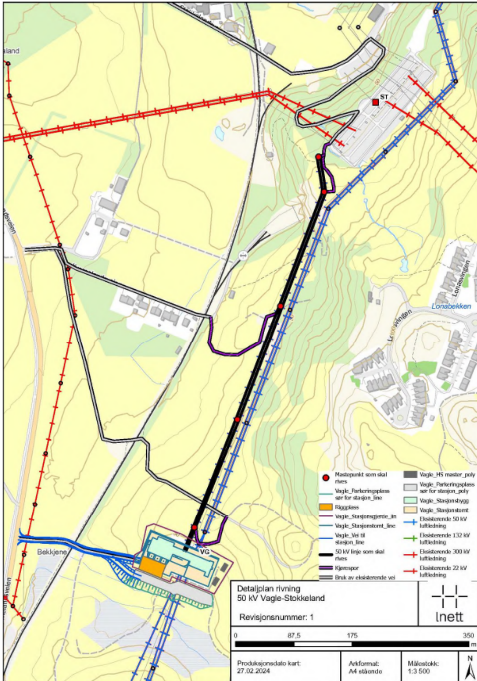
Figur 2: Detaljplankart for rivning av 50kV kraftledning mellom Vagle og Stokkeland transformatorstasjon. Grå linjer viser eksisterende vei, mens lilla linjer viser kjørespor, og røde punkter viser mastene som skal rives. Kilde: Lnett, 2024.
