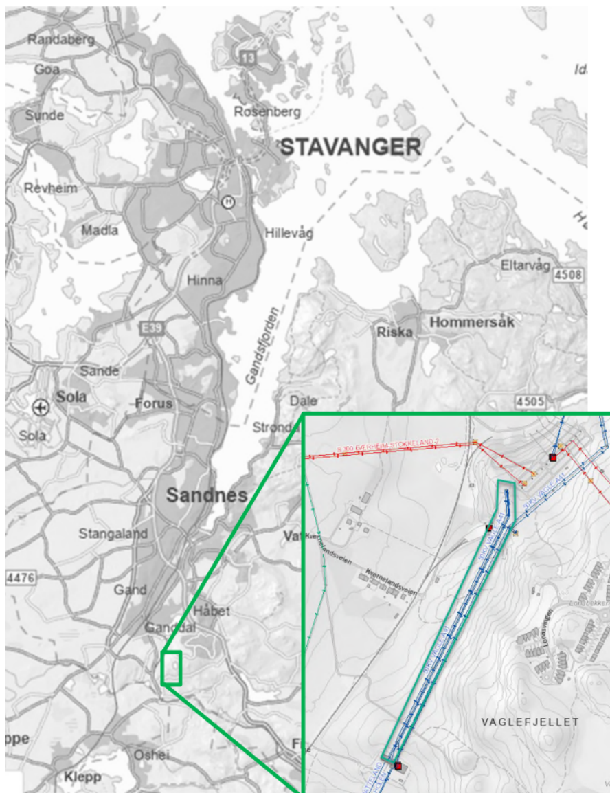
Figur 1: Oversiktskart med 50 kV kraftledningen mellom Stokkeland og Vagle som Lnett søker om å legge ned. Kilde: Lnett, 2024.
