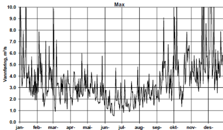
Figur 1-4. Plott som viser sesongvariasjon i maksimumsvannføringer gjennom året (døgndata). 15
