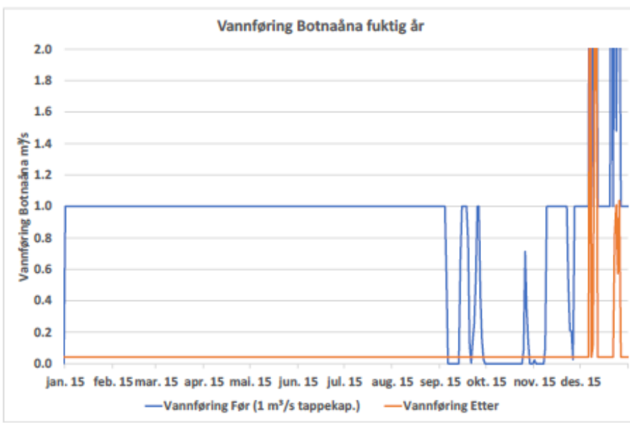
Figur 1-8. Plott som viser vannføringsvariasjoner i et vått (2020) år (før og etter utbygging). 19
