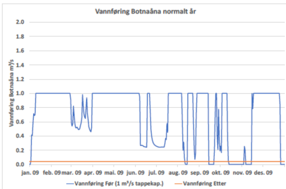
Figur 1-7. Plott som viser vannføringsvariasjoner i et middels (2009) år (før og etter utbygging). 18
