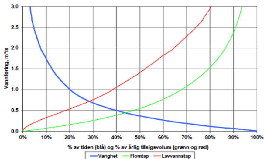
Figur 1-11. Varighetskurve, kurve for flomtap og for tap av vann i lavvannsperioden (år).
