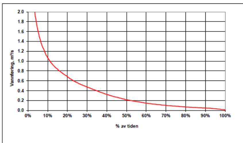
Figur 1-9. Varighetskurve for sommersesongen (1/5 – 30/9).
