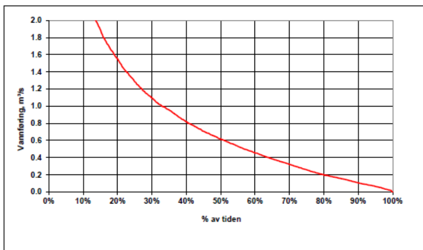
Figur 1-10. Varighetskurve for vintersesongen (1/10 – 30/4).
