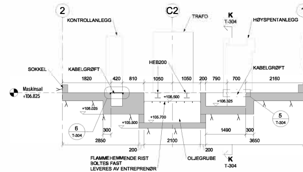
Snitt L-L 1 : 50
