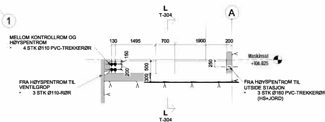
Snitt K-K 1 : 50
