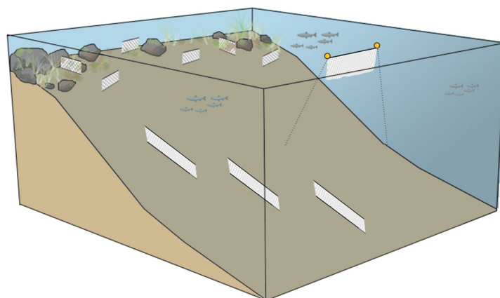
Figur 4.1. Skjematisk oppsett for bunngarnfiske med nordiske oversiktsgarn på hver garnstasjon iht. FIST-standard som benyttes i ØKOSTOR-programmet (Eikland mfl., 2022). Standard for fiske ved bunnen er seks enkeltgarn i strandsona og tre lenker á tre garn på dypere vann. Illustrasjon: Sigrd Skoglund, NINA.
