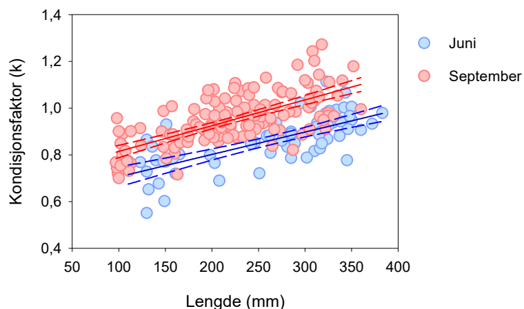
Figur 5.12. K-faktor mot lengde for 66 røye fanget i juni (blå sirkler) og 147 røye fanget i september (rød sirkler) under prøvefiske i Nesjøen i 2021. Blå og rød heltrukne linjer viser regresjonslinja for de to periodene, mens stiplede blå og røde linjer viser 95 % konfidensintervall til regresjonslinjene.
