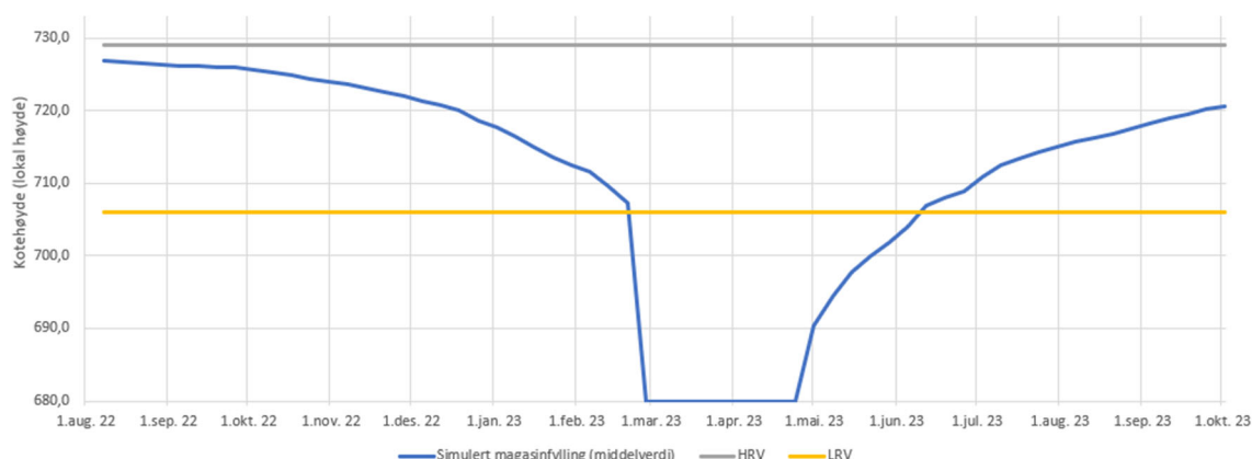
Figur 3.1. Plan for nedtapping av Nesjøen med middelerdi for estimert vannstand og simulert magasinifylling (blå strek) i perioden 1. august 2022 til 1. oktober 2023. Laveste og høyeste regulerte vannstand er markert ved hhv. gul og grå horisontal linje. Kilde: Statkraft.
