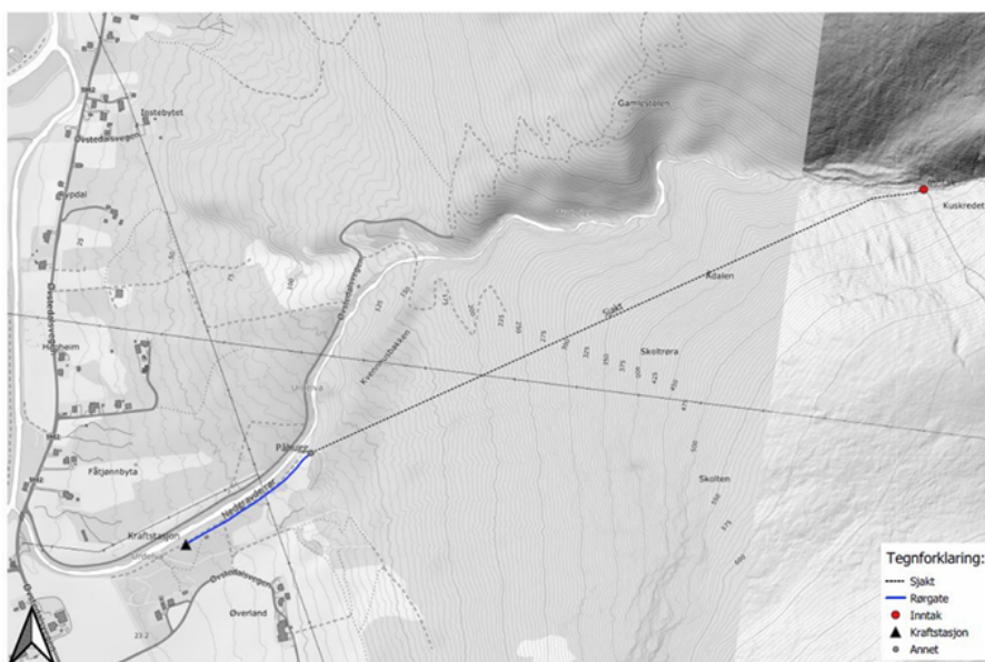
Figur 13: Revidert plan for Urdelva kraftverk (2025). Rørgata er lagt på østsiden av elva for å unngå edellauvskog og kulturminner på vestsiden. Kraftstasjonen er plassert høyt opp i elva, over en naturlig fiskestopp, slik at hensynet til anadrom fisk blir ivarettatt. Denne løsningen reduserer samtidig konfliktene med naturmangfold og kulturmiljø, og følger opp innspillene fra tidligere høringsrunder.
