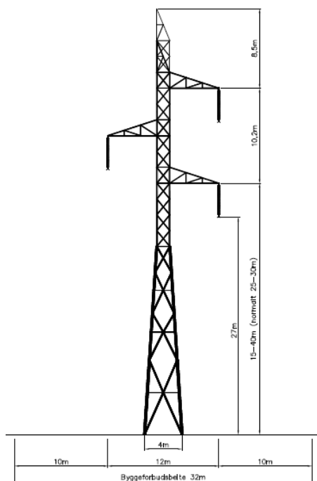
Figur 13 Vurderte alternative masteutforminger i bratt terreng. Statnett Tårnmast 420 kV, med et byggeforbudsbelte på ca. 32 meter mot 40 meter normalt.
