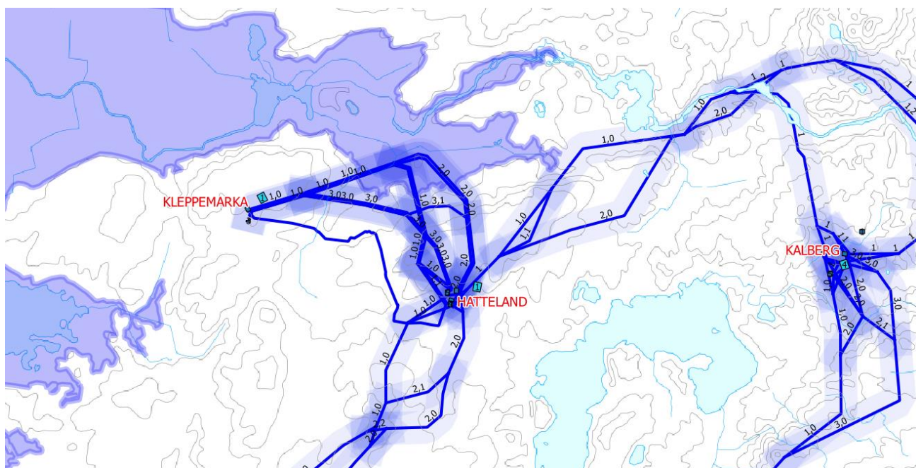
Figur 222. Figgjoelva i steinalderen med 10 m (lilla) høgare havnivå. (Rådgjevande Arkeologar 2016).
