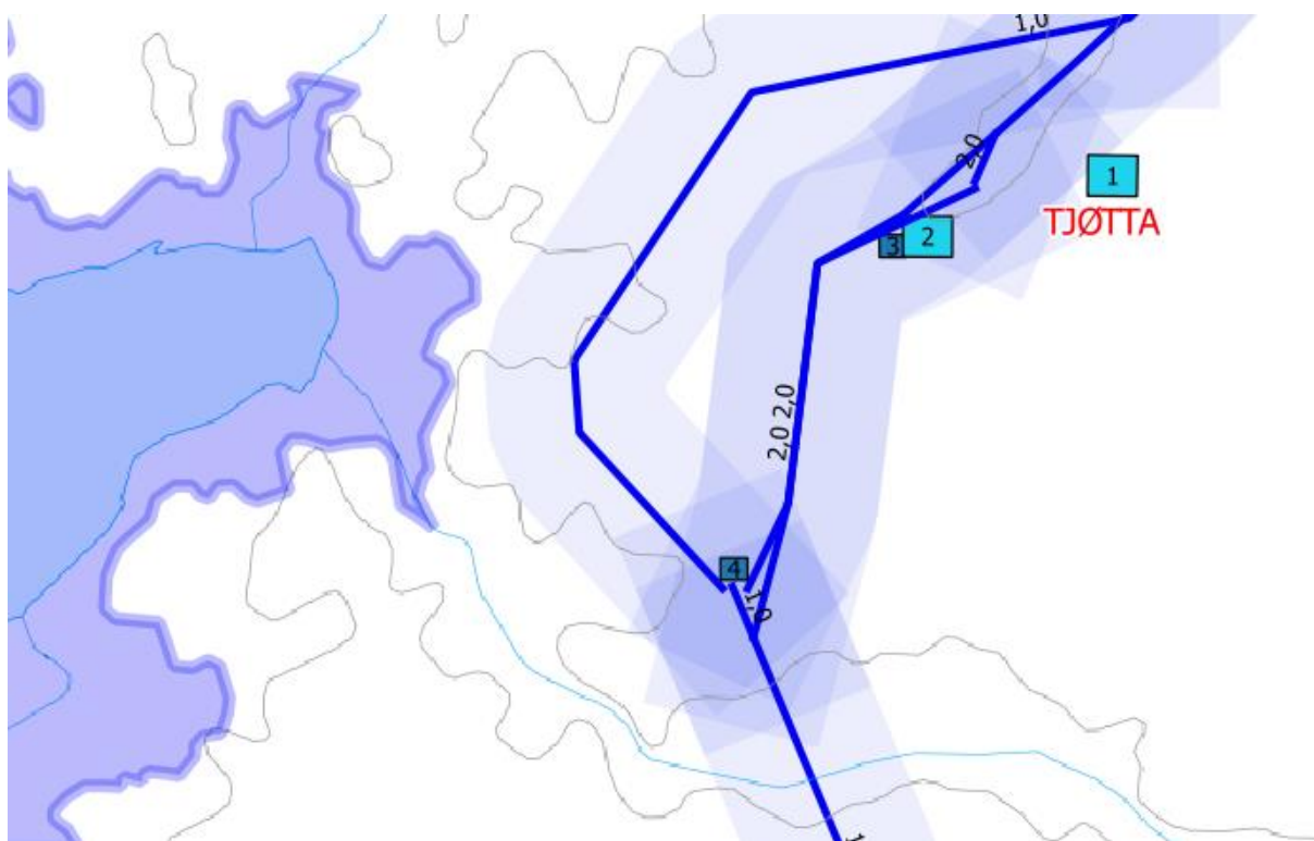
Figur 223. Horpestadvatnet i steinalderen med 10 m (lilla) høgare havnivå. (Rådgjevande Arkeologar 2016).
