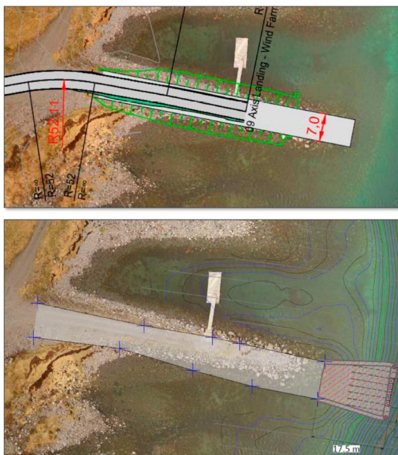
Figur 2. Opprinnelig plan (øverst) og revidert plan (nederst). Figur hentet fra søknaden av 06.10.2021.
