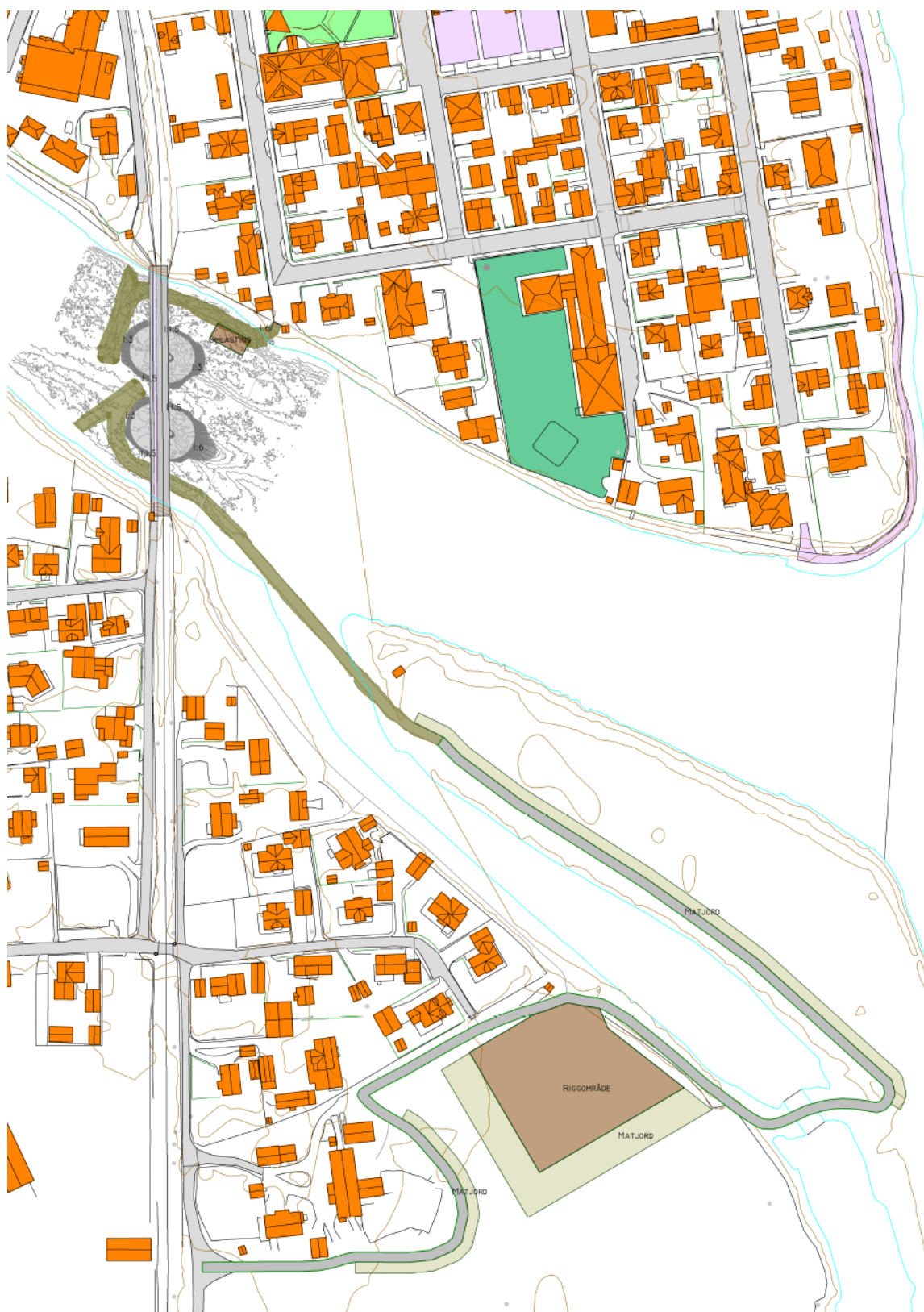
Figur 2-1. Skjematisk skisse over planlagt erosjonssikring og midlertidige anleggsveger. Merk at sikring av elvbredde nedstrøms tiltaket ikke er vist i denne skissen.
