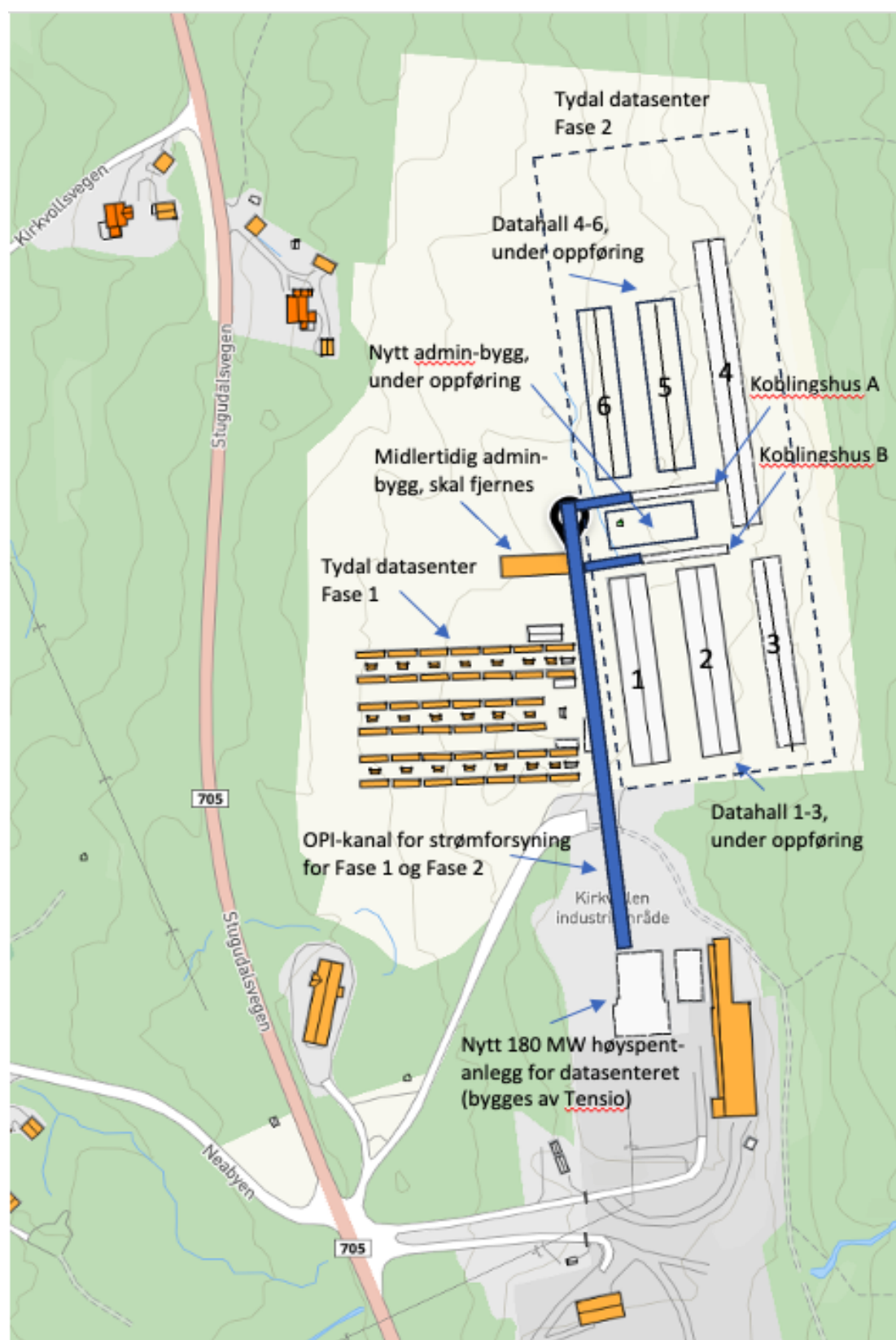
Situasjonsplan for koblingsanlegg for Fase 2 og OPI-kanal for tilkobling til Tensio
