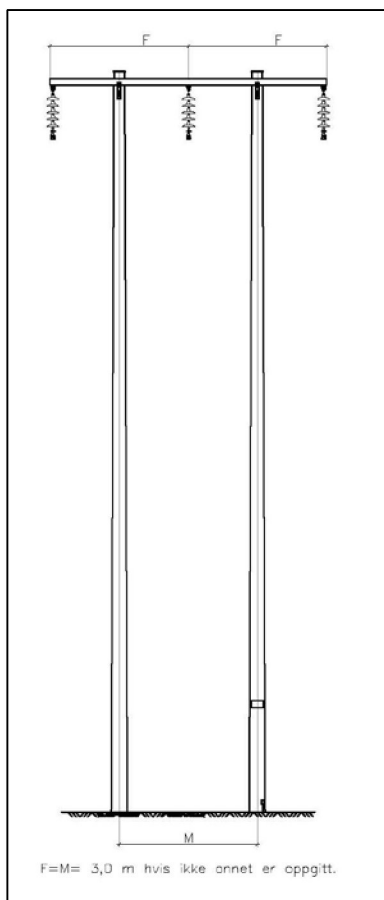
Figur 6. Mastebilde for bæremast. Kilde: Jøsok Prosjekt AS.
