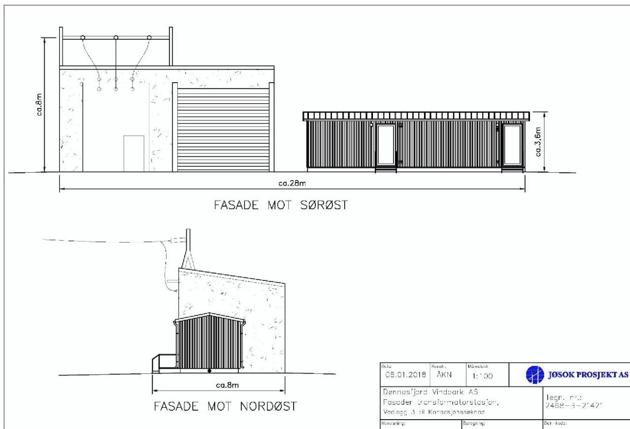
Figur 5. Fasade på trafo og servicebygg (foreløpig skisse). Kilde: Jøsok Prosjekt AS.
