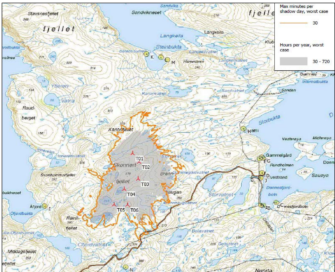
Figur 25. Skyggekast (worst case) og bebyggelse. Kilde: Enercon (2018).
