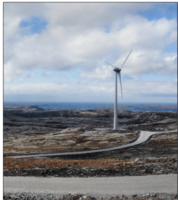
Figur 20. Minst mulig eksponering av kranoppstillingsplass og fundament er viktig for god landskaps-tilpassing, her vist ved senking av oppstillingsplass slik at utstrakte fyllinger unngås og gjenstående knauser delvis skjermes for innsyn.
