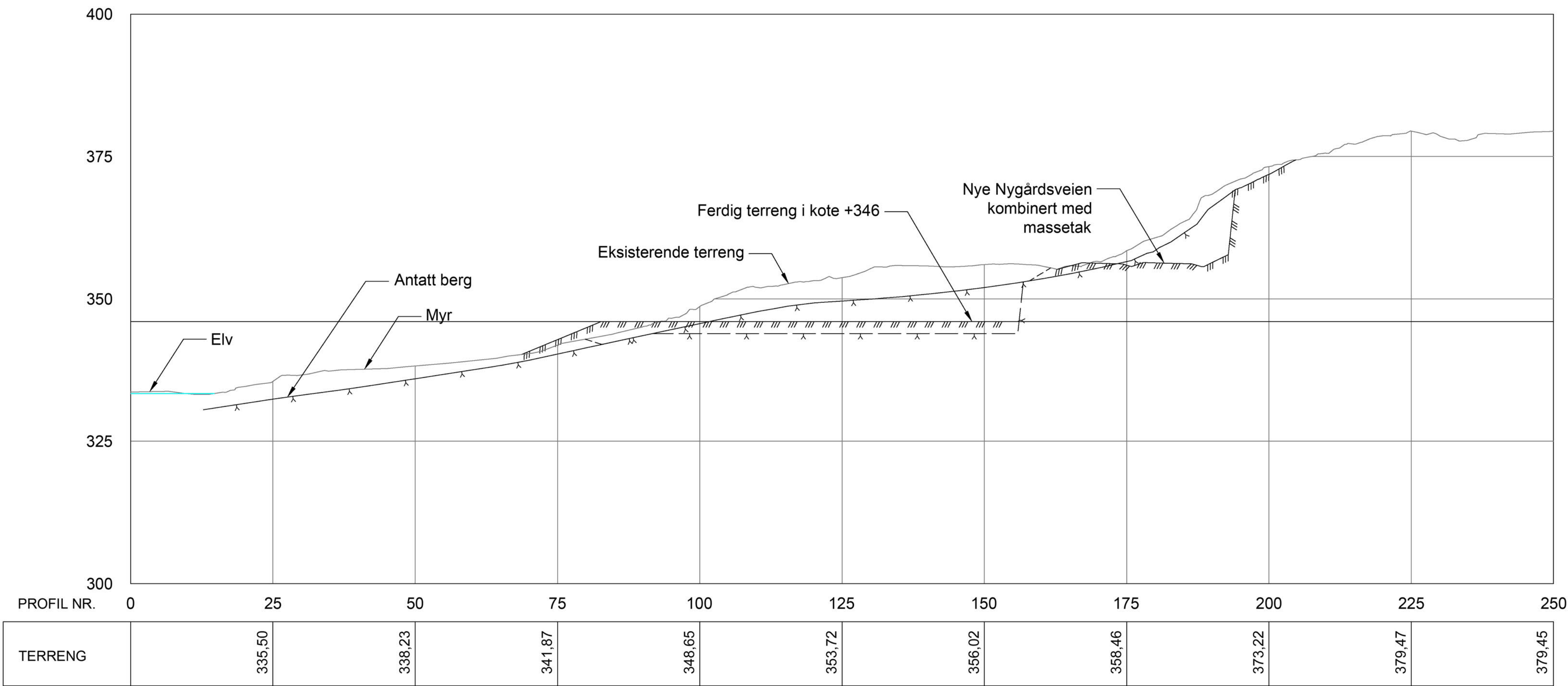
Tverrsnitt 1:500
