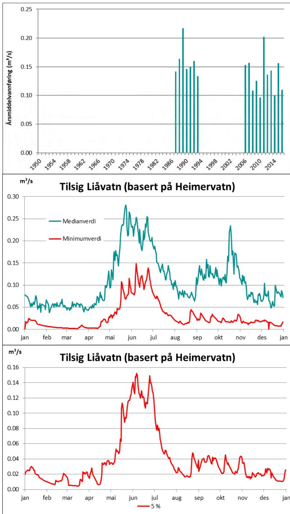
Figur 3-2 Flerårsstatistikk for tilsig til Liåvatn, basert på NVE-måleserie Heimervatn.
