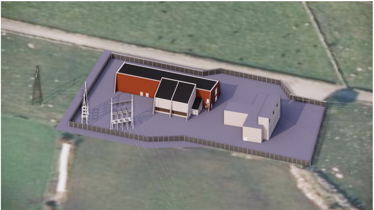
Figur 4 Hatteland transformatorstasjon, sett fra øst
