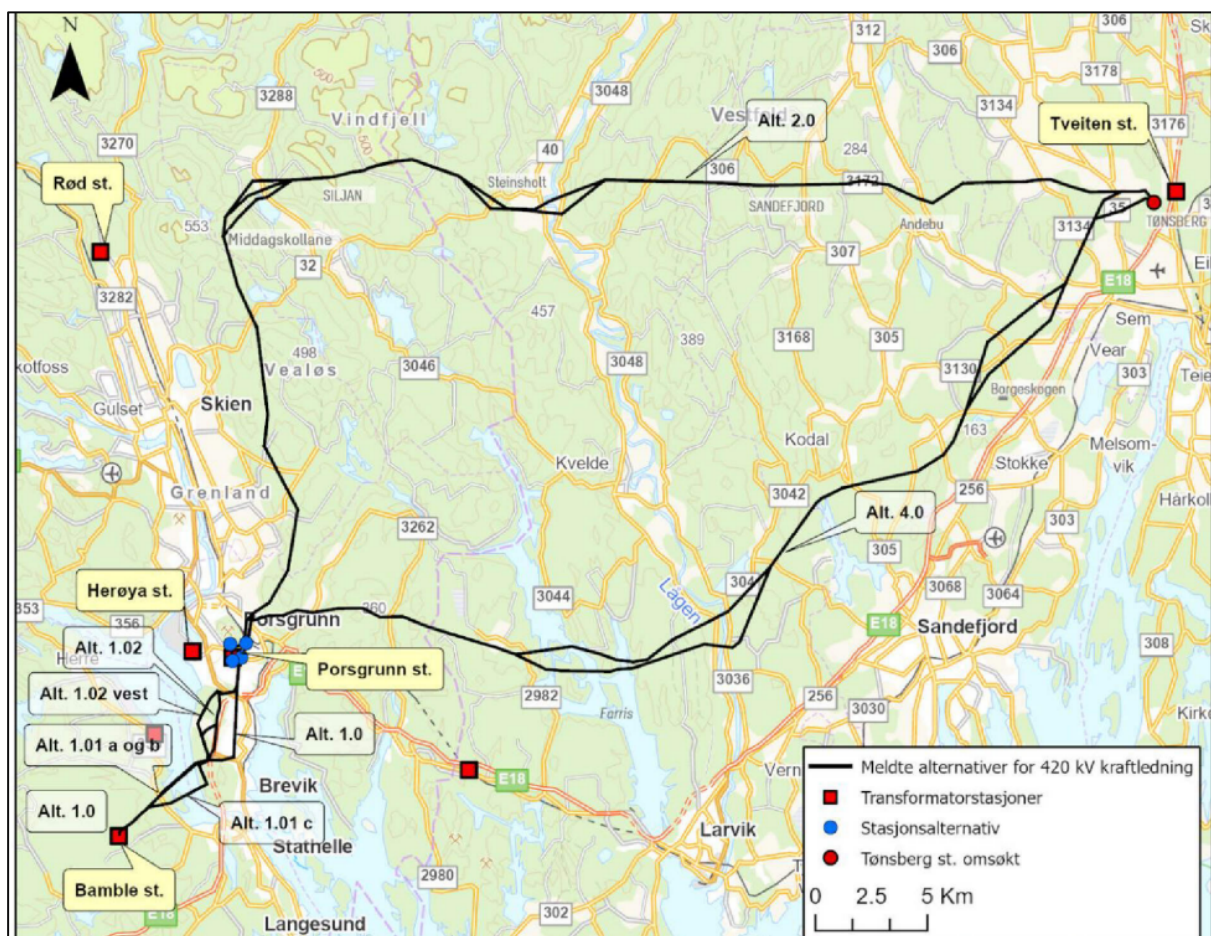
Figur 1. Alternativer for 420 kV forbindelse mellom Bamble, Porsgrunn og Tønsberg transformatorstasjon. Meldte alternativ og varianter er markert med svart strek. Hentet fra Statnetts melding.
