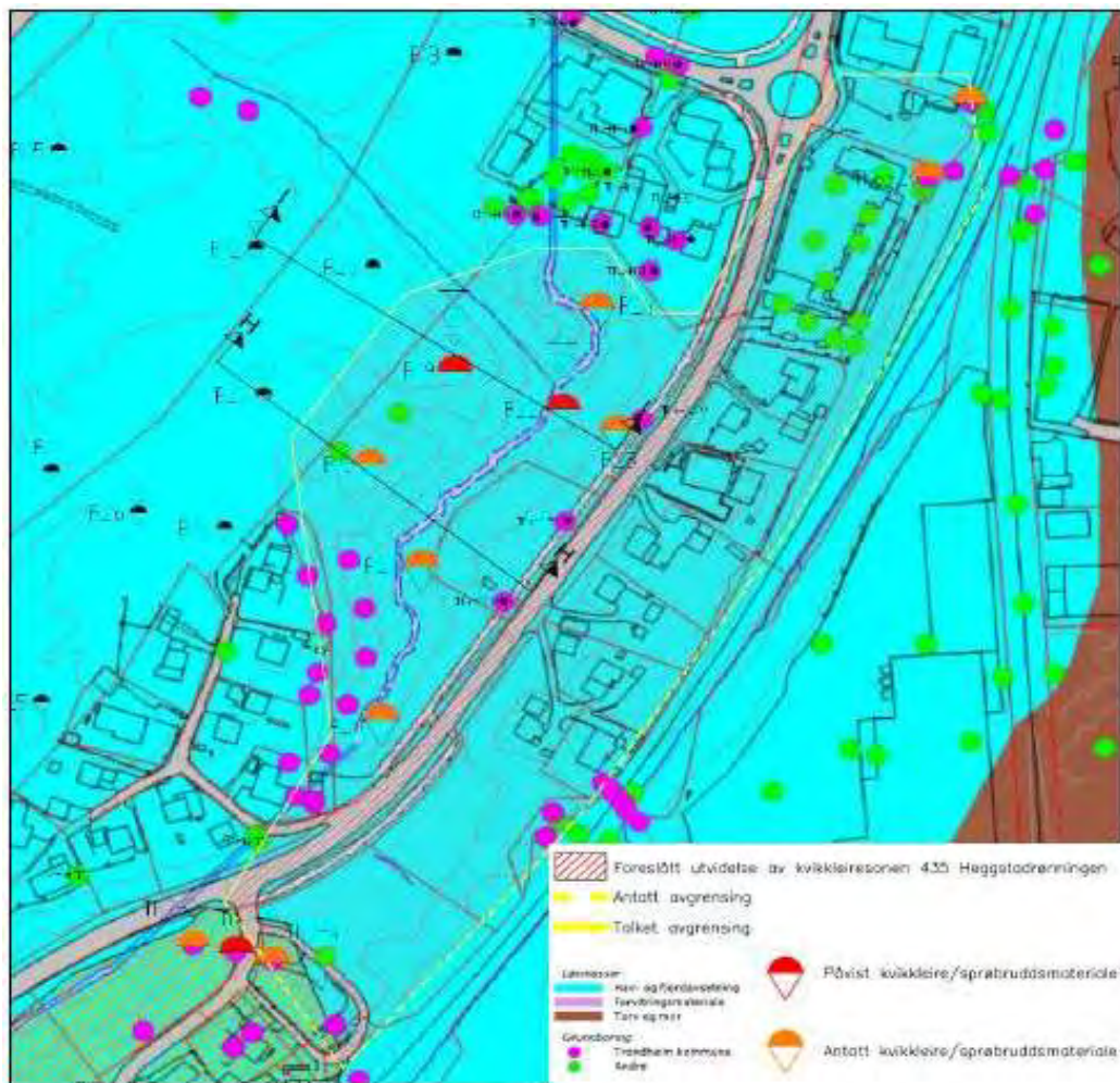
Figur 1 - Utdrag fra tegning 415342.2-RIG-TEG-002 REV A, situasjonsplan som viser foreslått avgrensning av kvikkleiresone
