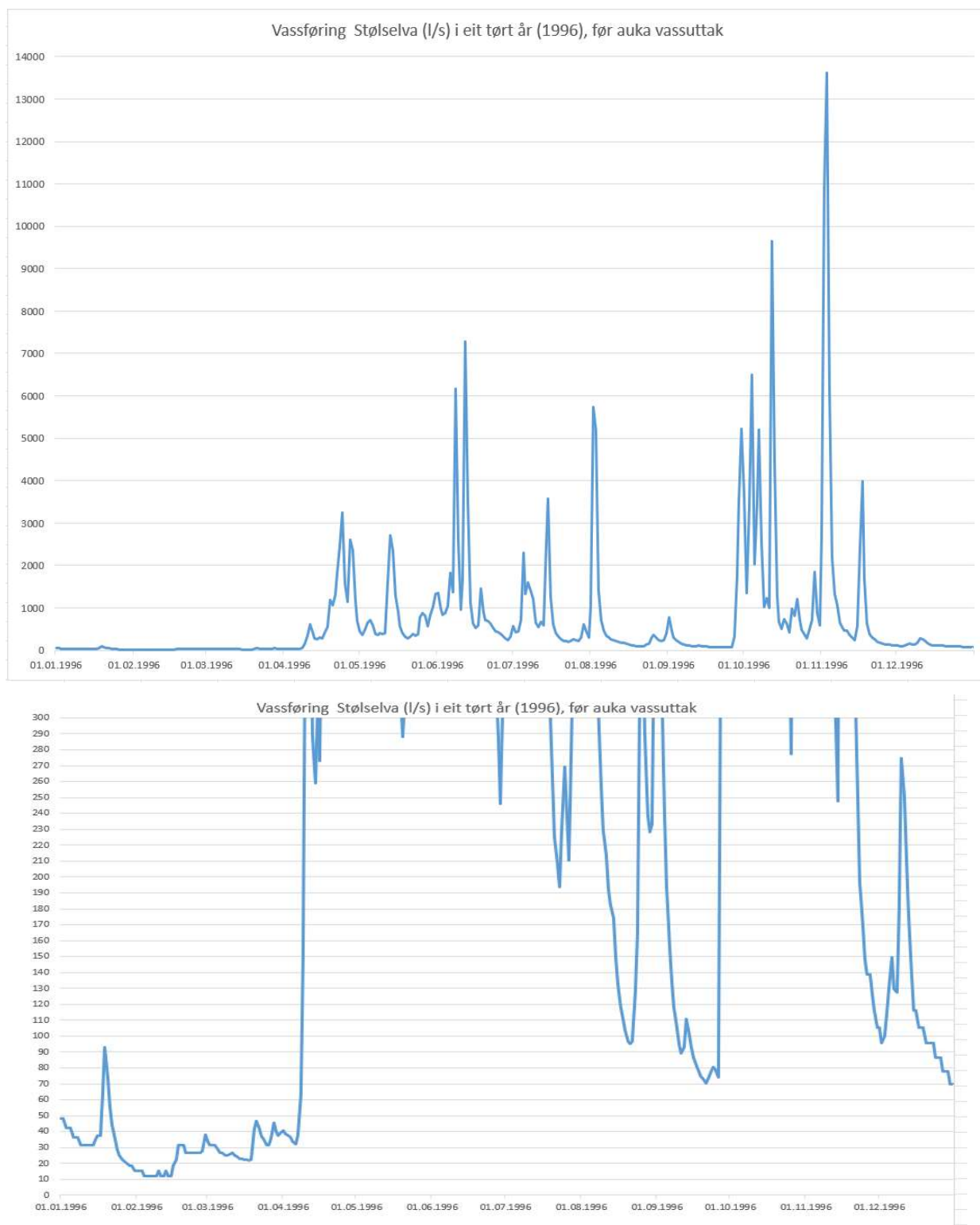
Figur 6. Plott som viser vassføringsvariasjonar i eit tørt (1996) år (før og etter utbygging). 17
