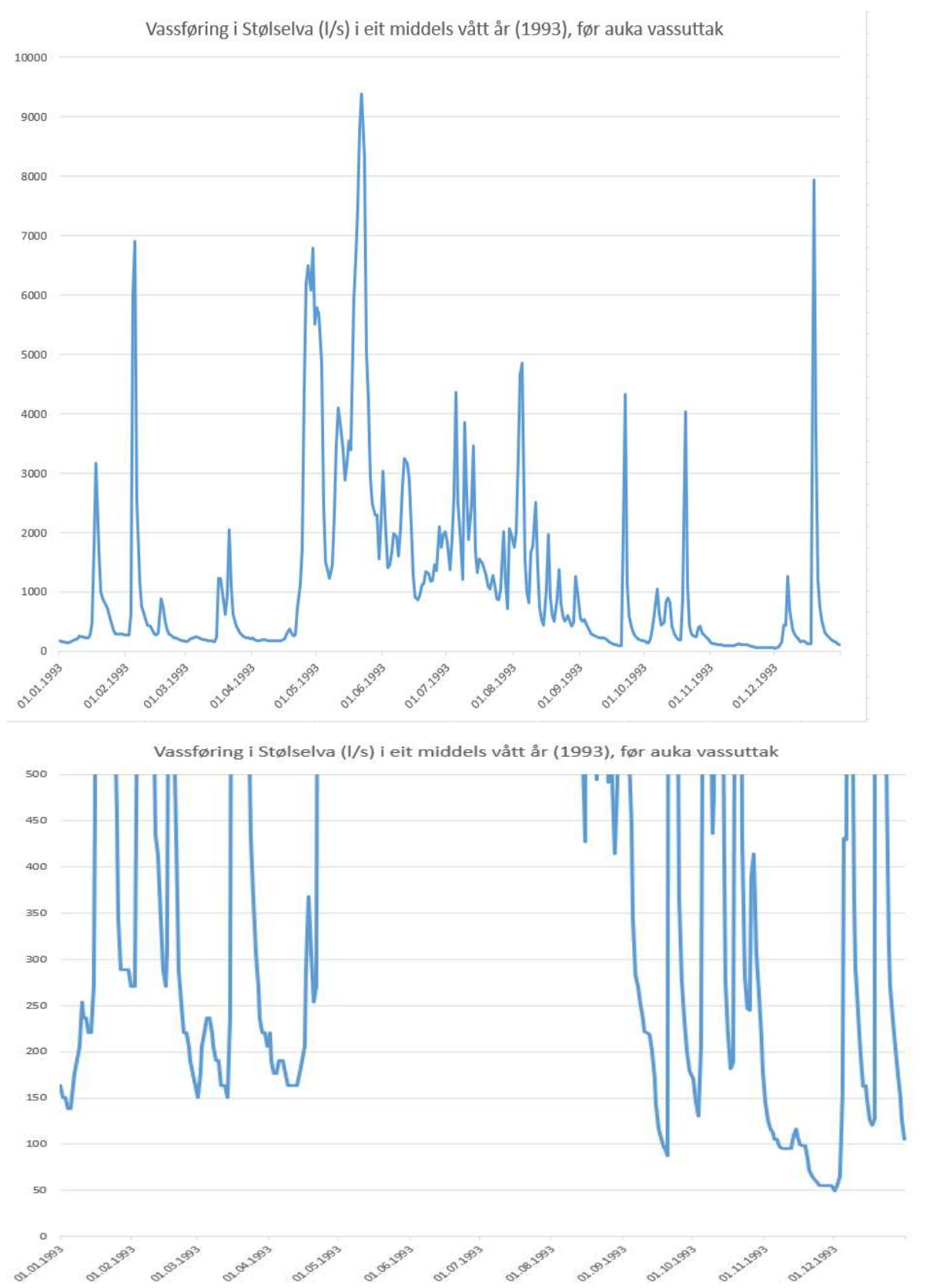
Figur 7. Plott som viser vassføringsvariasjonar i eit middels (xxxx) år (før og etter utbygging). 18
