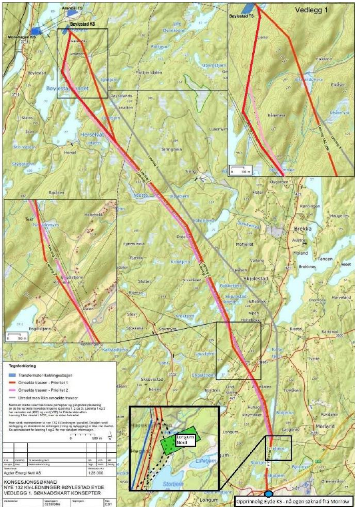
Figur 1: Plassering av ny 132 kV Bøylestad–Eyde og ny Longum Nord transformatorstasjon.
