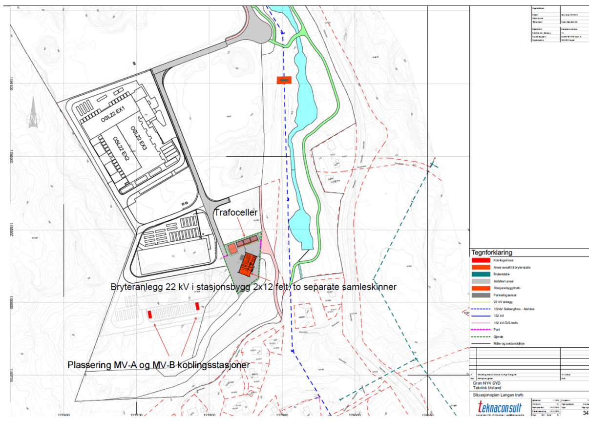
Kart 1: Situasjonsplan som viser plassering av trafoceller, bryteranlegg og koblingsstasjoner. Kilde: Green Mountains søknad av 1.juli 2025.
