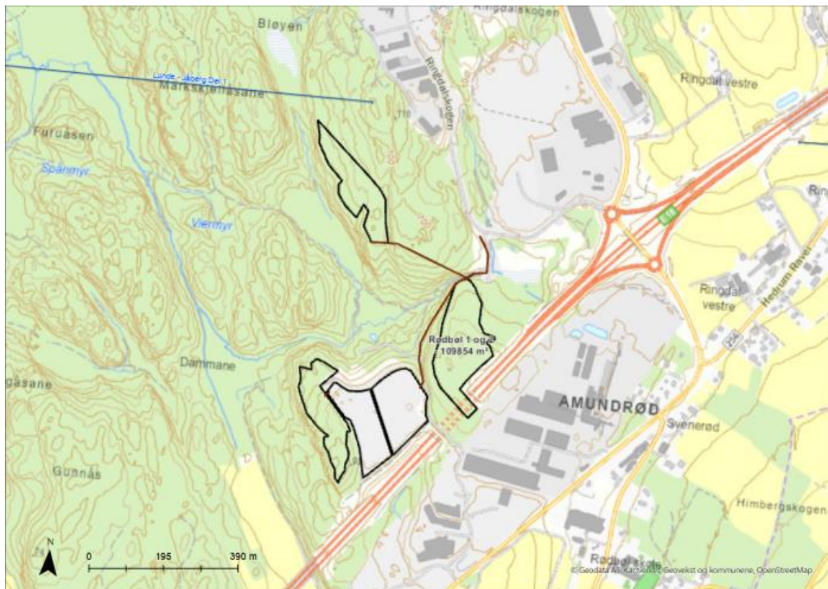
Figur 2-2: Oversikt over tiltaksområdet. Planlagt tilknytningstrasé for solkraftverket med ny 22 kV jordkabeltrasé vist med brun linje.
