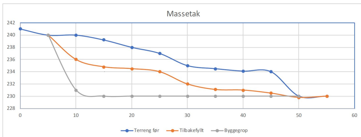
Figur 5: Eksempel på profil som viser opprinnelig terreng, byggegrup og tilbakefylt terreng. Eksemplet er hentet fra Statnetts håndbok i terrengbehandling (2024).
