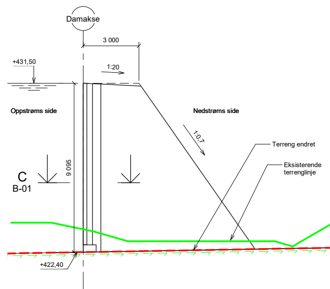
Snitt A-A 1 : 100
