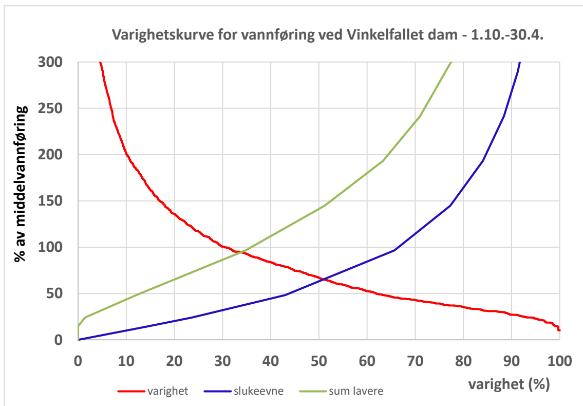
Figur 10. Varighetskurve for vintersesongen (1/10 – 30/4). Middelvannføring vinter 2,07 m 3 /s.
