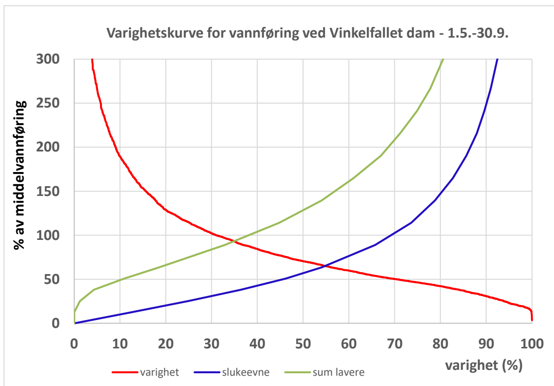
Figur 9. Varighetskurve for sommersesongen (1/5 – 30/9). Middelvannføring sommer 7,88 m 3 /s.
