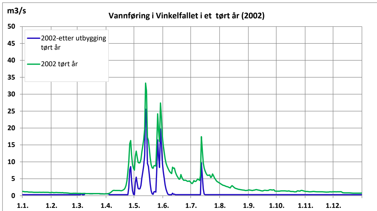
Figur 6. Plott som viser vannføringsvariasjoner i et tørt (2002) år (før og etter utbygging). 17
