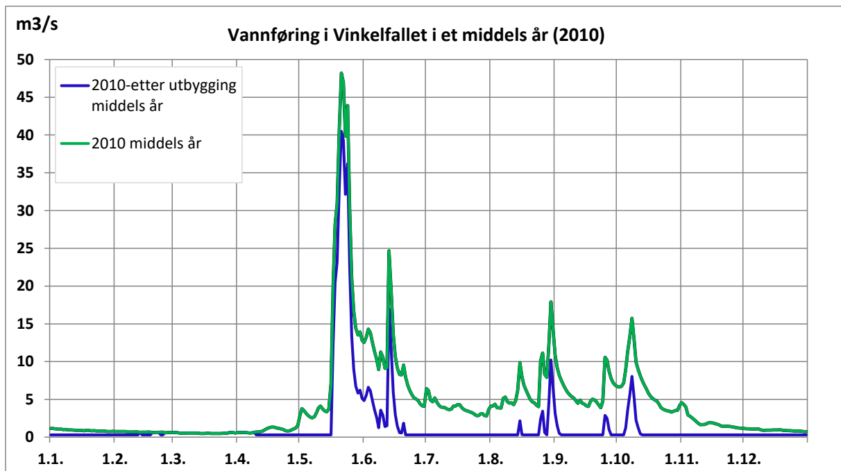
Figur 7. Plott som viser vannføringsvariasjoner i et middels (2010) år (før og etter utbygging). 18
