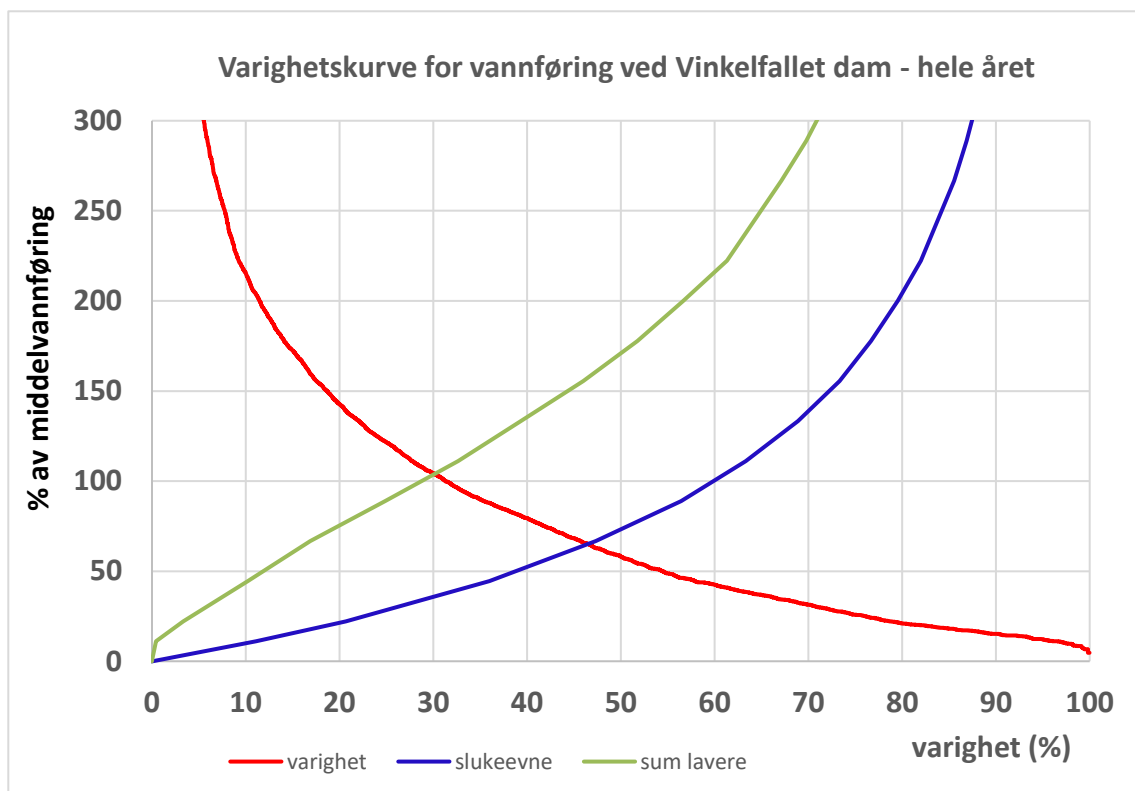
Figur 11. Varighetskurve, kurve for flomtap og for tap av vann i lavvannsperioden (år). Middelvannføring 4,50 m 3 /s.
