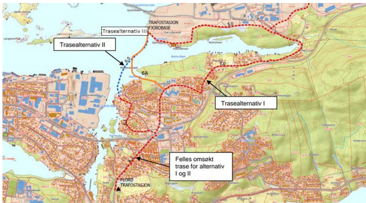
Figur 2: syner omsøkte kabeltrasear frå Botnaneset trafostasjon til Florø trafostasjon.
