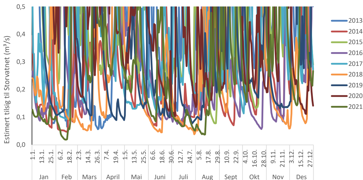
Figur 7. Estimert avrenning til Storvatnet gjennom året for perioden 2013-2021. Vannføringer over 0,5 m³/s vises ikke i figuren.
