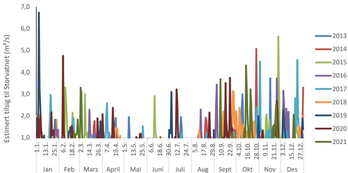
Figur 6. Estimert avrenning til Storvatnet gjennom året for perioden 2013-2021. Vannføringer under 1 m³/s vises ikke i figuren.
