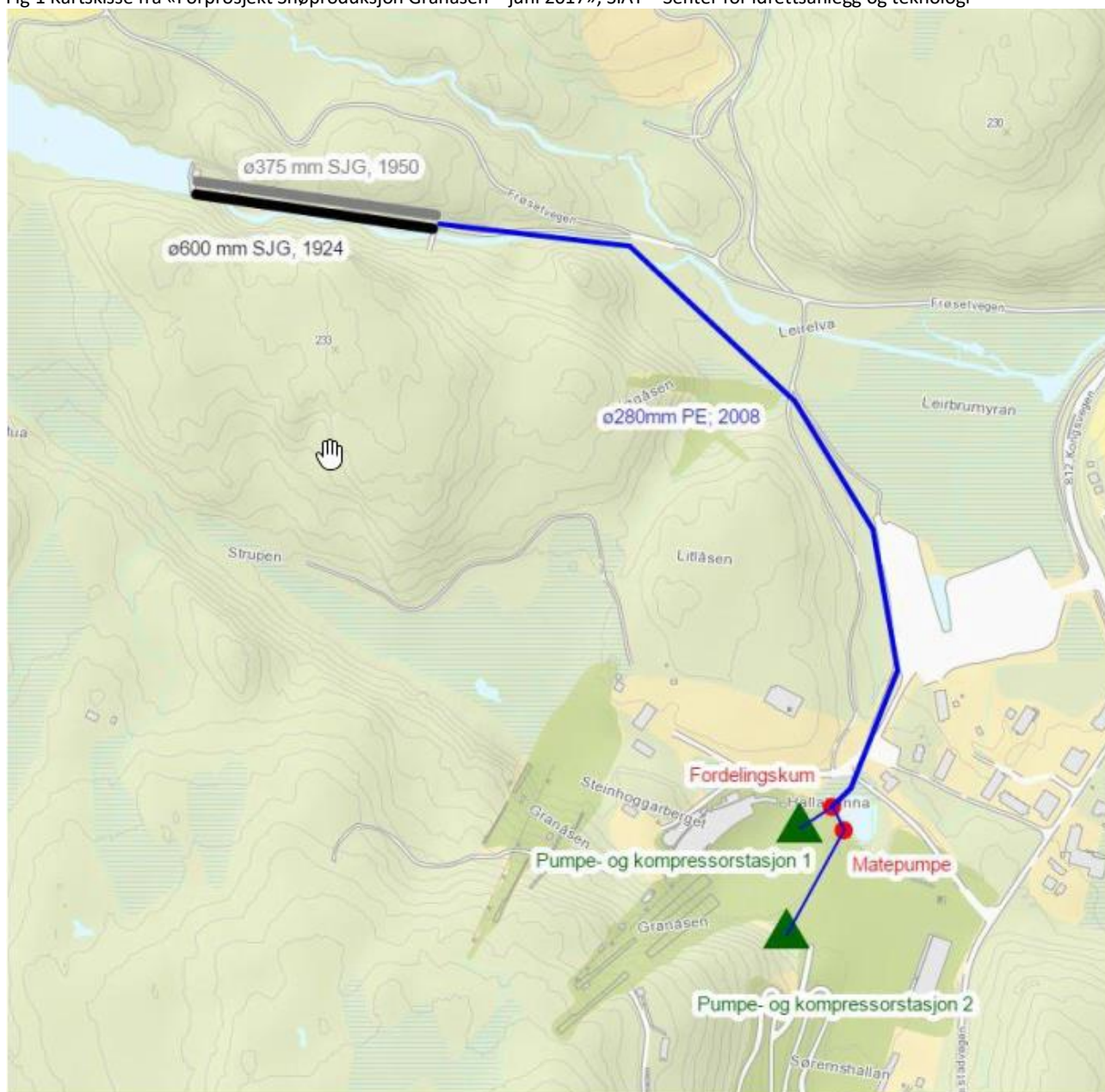
Fig 1 Kartskisse fra «Forprosjekt Snøproduksjon Granåsen – juni 2017», SIAT – Senter for idrettsanlegg og teknologi
