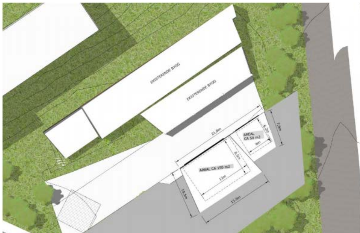
Figur 11 – Plantegning Fornebu transformatorstasjon
