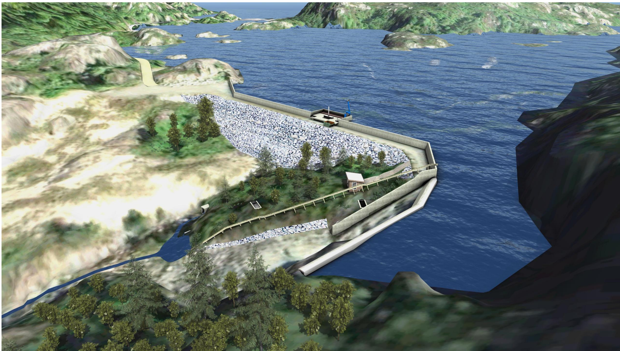
Fotoillustrasjon: Dam og inntak Honnefoss. Oversiktsbilete mot nordaust. Nytt lukehus midt i bildet
