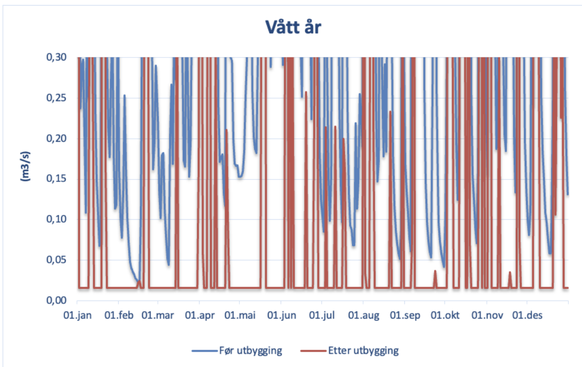
Figur 8. Plott som viser vannføringsvariasjoner i et vått (2017) år (før og etter utbygging). 19
