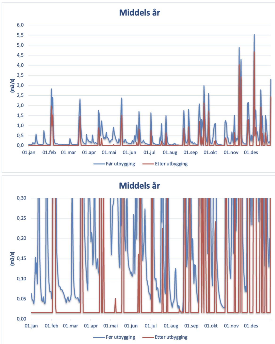
Figur 7. Plott som viser vannføringsvariasjoner i et middels (2004) år (før og etter utbygging). 18
