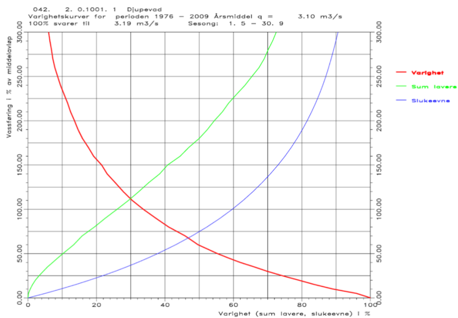
Figur 9. Varighetskurve for sommersesongen (1/5 - 30/9).
