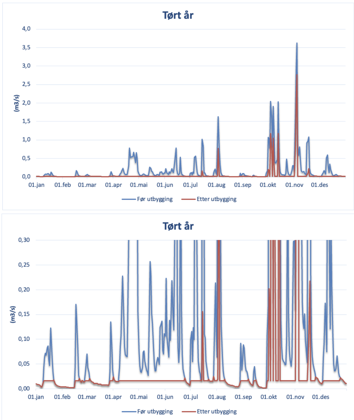
Figur 6. Plott som viser vannføringsvariasjoner i et tørt (1996) år (før og etter utbygging). 17
