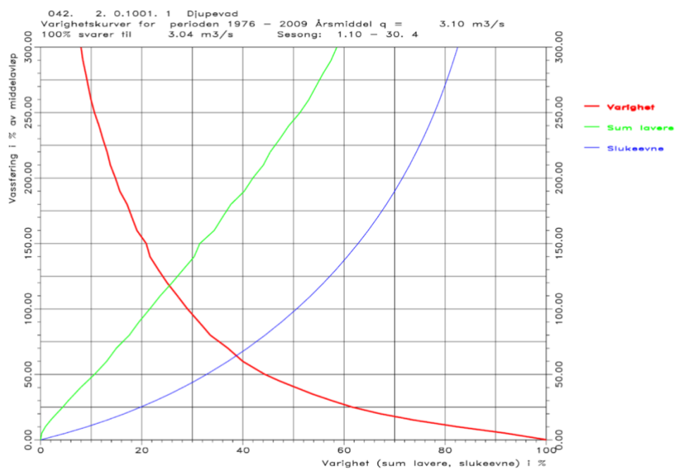
Figur 10. Varighetskurve for vintersesongen (1/10 - 30/4).
