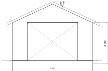
FASADE VEST 1 : 50
