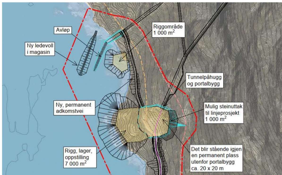
Illvatn pumpekraftverk - portalbygg
