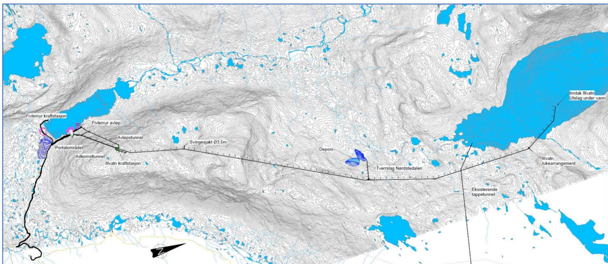
Illvatn kraftverk
