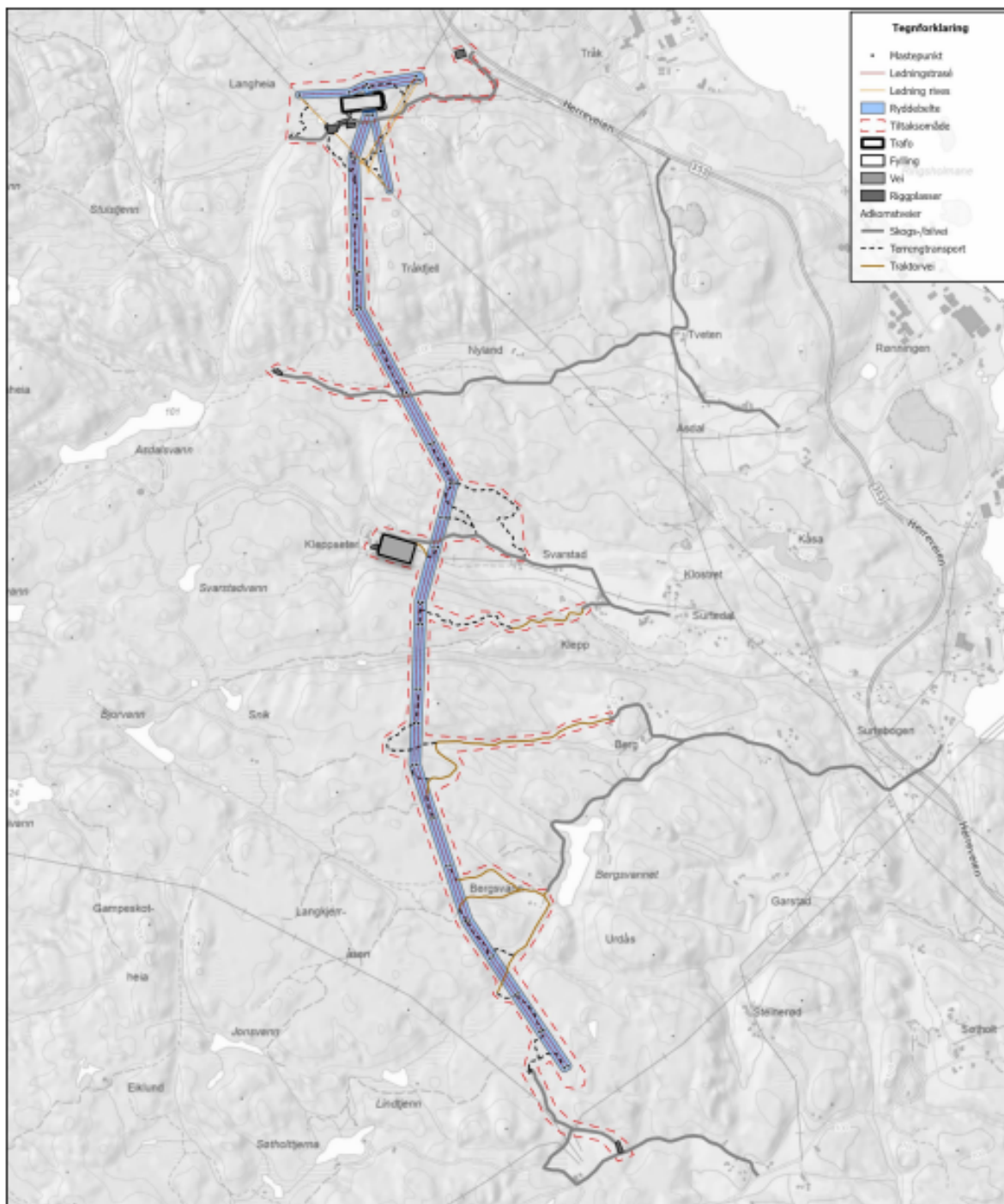
Figur 1: Oversikt over tiltaket. Frier transformatorstasjon er vist med lys rektangel nord for Tråkfjell. Traseen for 132 kV luftledning er vist i blått. Tiltaksområdet er markert med rød stiplet strek.
