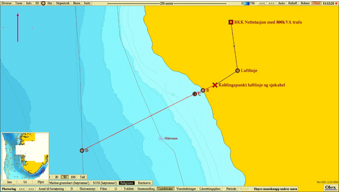
Bilde av trasé for 22 kV sjøkabelen.
