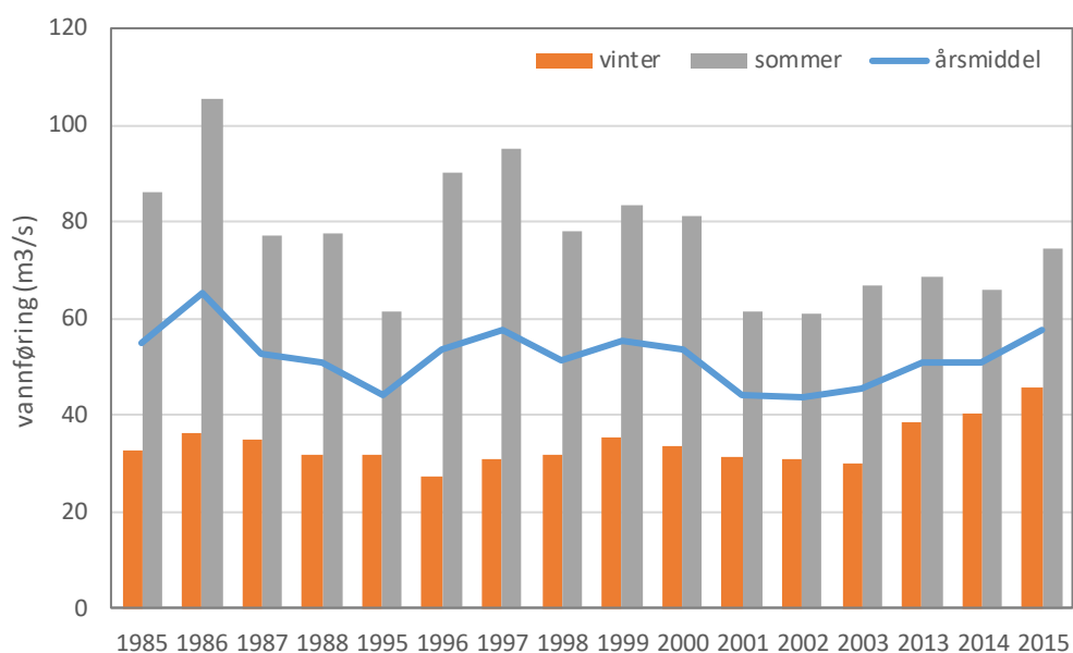
Figur 7. Midlere vannføringer ved Lavika i perioden 1985-2015.
