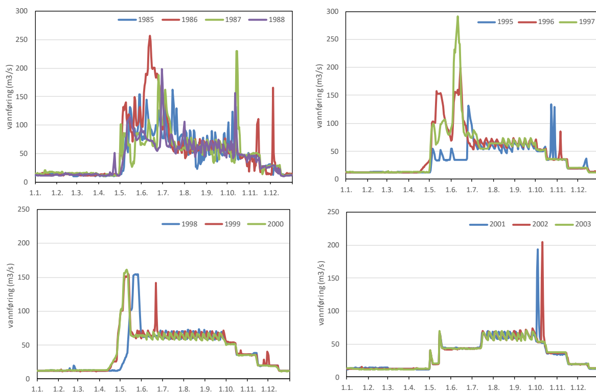
Figur 4. Midlere vannføring i Suldalslågen ved Stråpa i periodene 1985-88, 1995-1997, 1998-2000 og 2001-2003.
