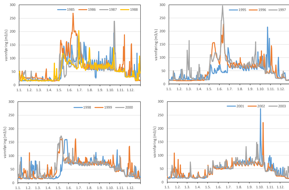
Figur 5. Midlere vannføring i Suldalslågen ved Lavika i periodene 1985-88, 1995-1997, 1998-2000 og 2001-2003.
