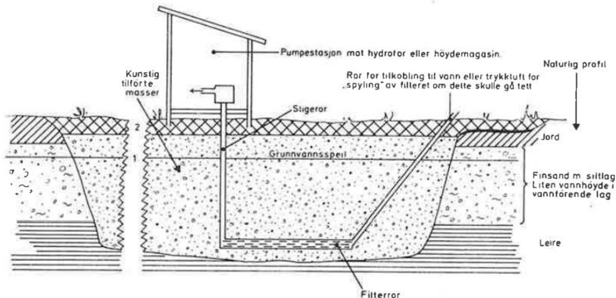
Figur 23 Gravd, horisontal brønn med masseutsifting (Huseby og Klemetsrud, 1980: Beskrivelse til vannressurskart Grunnvann i løsavsetninger: Hønefoss. Hydrogeologisk seksjon, spesiell rapport nr 19).
