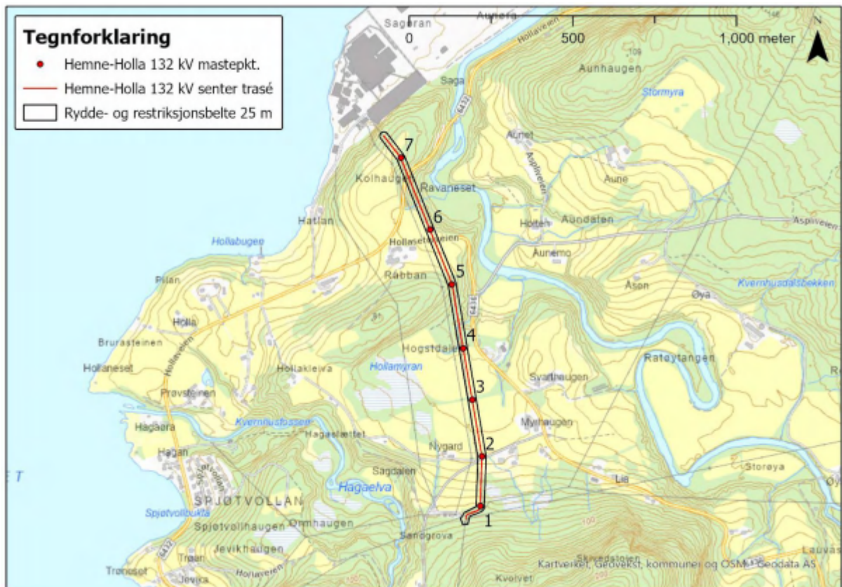
Figur 1: Oversiktskart ny 132 kV kraftledning mellom Hemne og Holla (Tensio)
