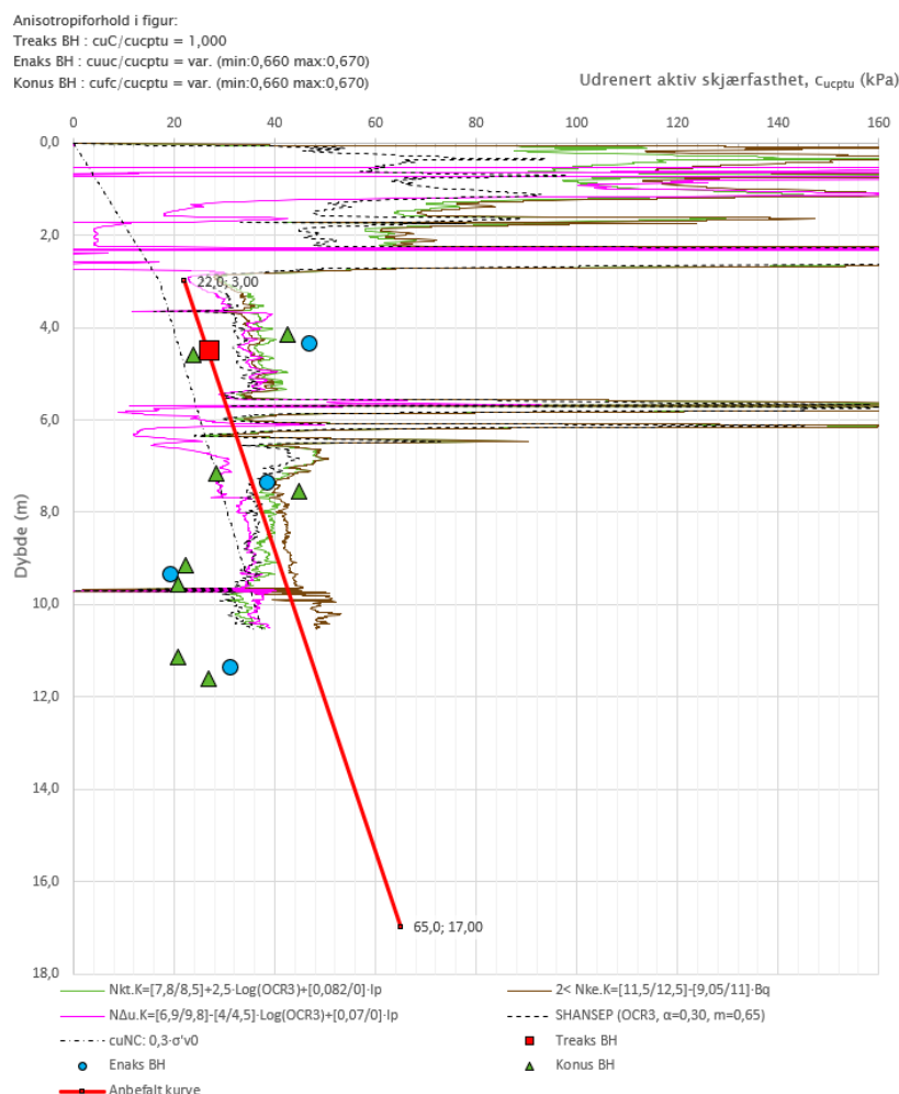
Figur 1 Designprofil for C_u basert på laboratorieundersøkelser i borhull NO_73 og trykksondering i borhull NO_104.
