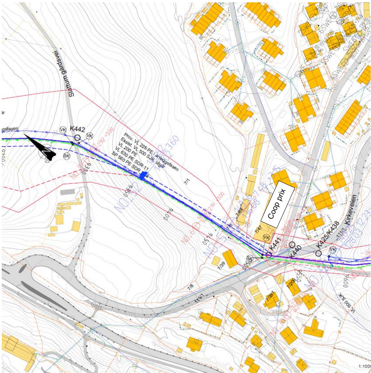
Figur 55 Plantegning med VA-trase og aktuelle borpunkt
