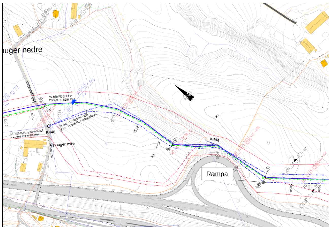
Figur 42 Plantegning med va-trase med aktuelle borpunkt
