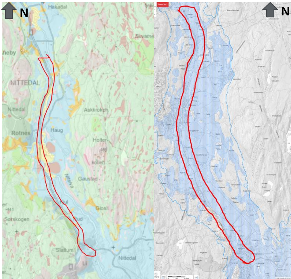
Figur 2 Løsmassekart til venstre og områder med mulighet for sammenhengende forekomst av marin leire til høyre. VA-trase ligger innenfor område skissert med rødt.
