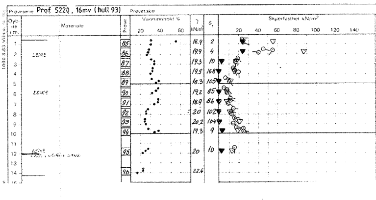
Figur 31: Utklipp fra prøveanalyse i posisjon C720B-93. Denne viser kvikkleire i dybdesjiktet 4-9 m (tilsvarer kt. +110,7 til +105,7), [13]
