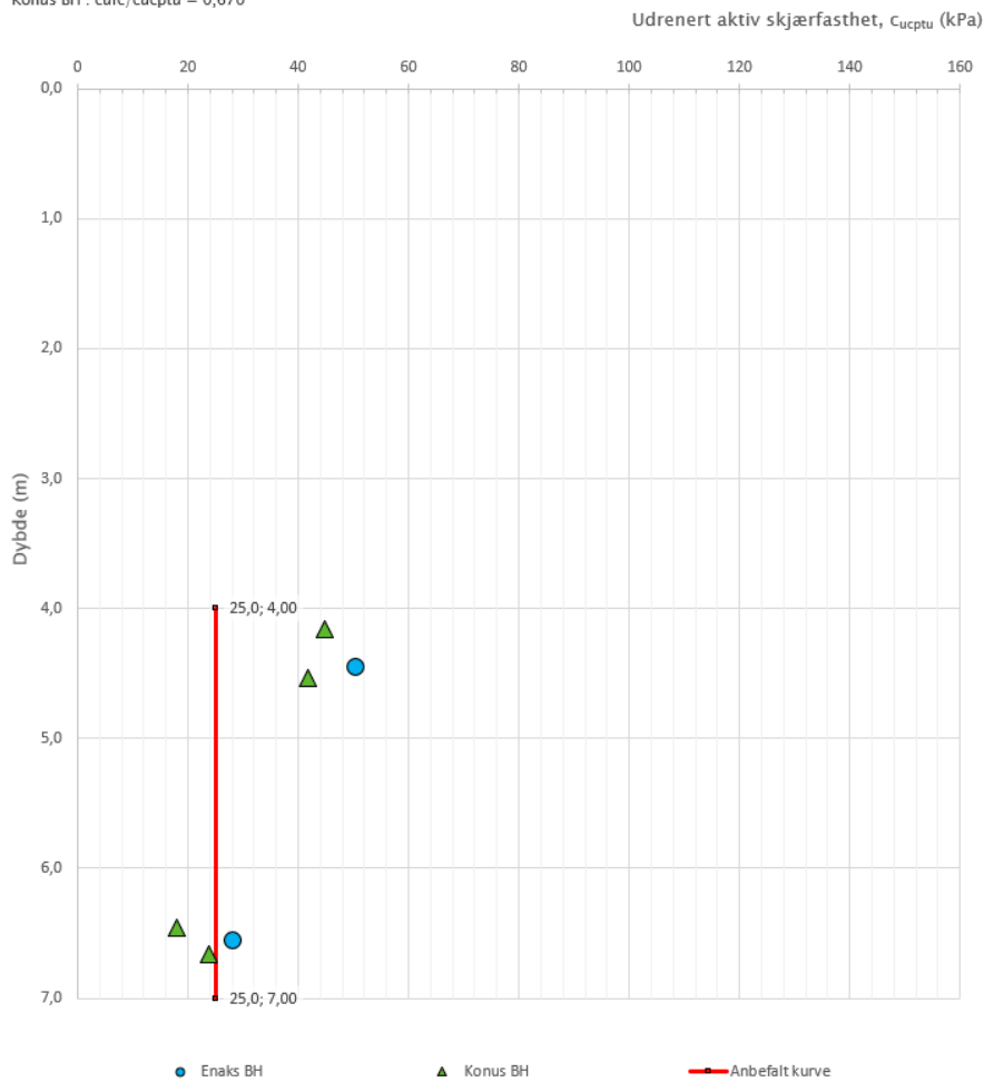
Figur 10 Designprofil for Cu basert på laboratorieundersøkelser gjennomført i borhull NO_13.
