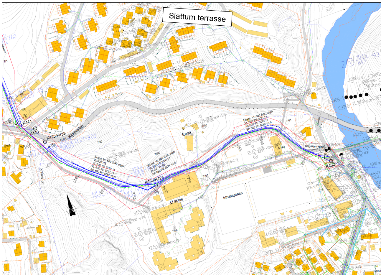
Figur 58 Plantegning med va-trase og aktuelle borpunkt.
