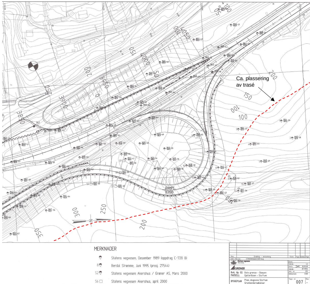
Figur 46: Utklipp fra tegning 007, [7], med ca. angivelse av VA-trasé.
