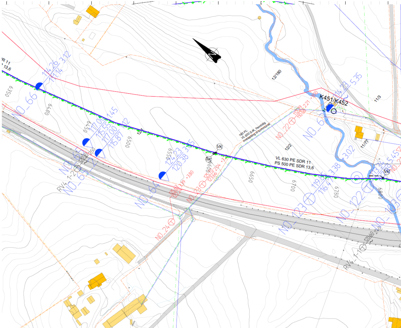
Figur 24 Plantegning med va-trase og aktuelle borpunkt.
