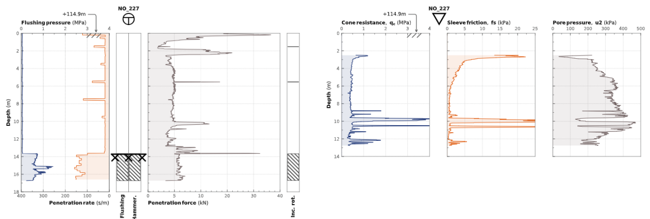
Figur 30: Sonderingsprofiler fra supplerende grunnundersøkelser i borpunkt NO_227
