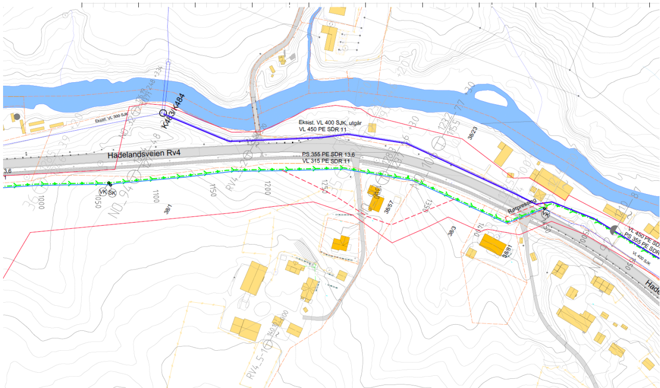
Figur 9 Plantegning med VA-trase og aktuelle borpunkt
