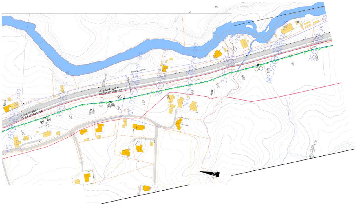
Figur 7 Plantegning med va-trase og aktuelle borpunkter
