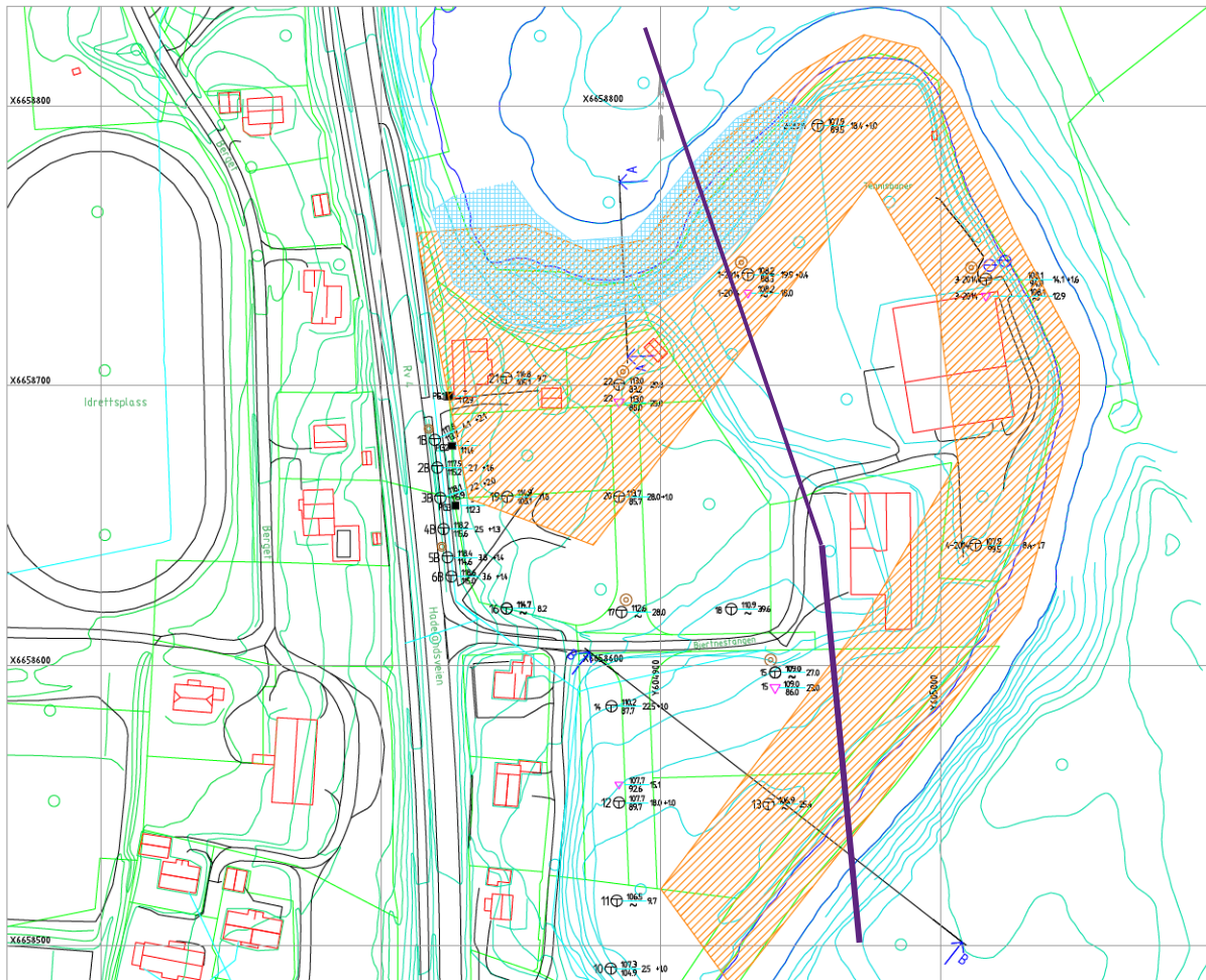
Figur 16 Faresone middels markert med oransje og erosjonssikring vist i blått [1]. Skissert va-trase vist med lilla strek
