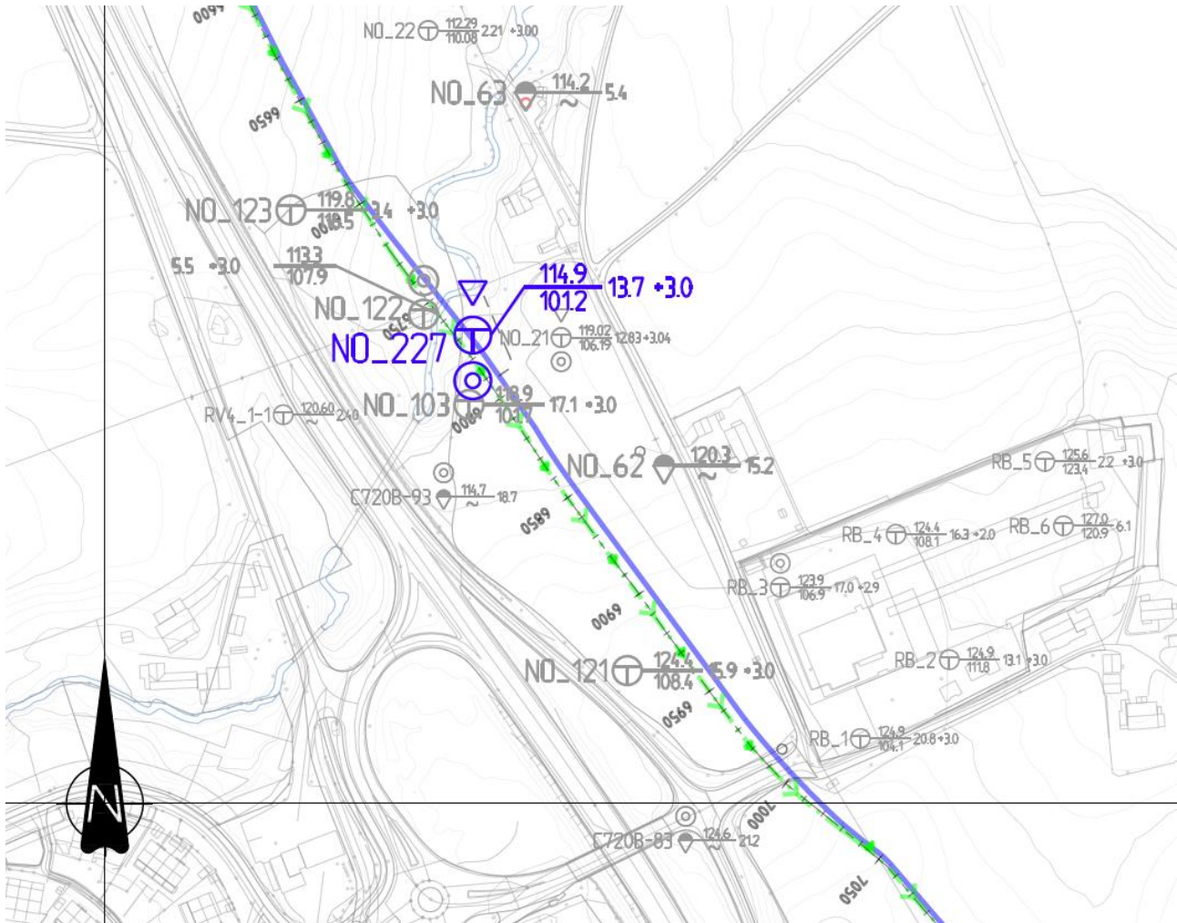
Figur 27 Plantegning med VA-trasé
