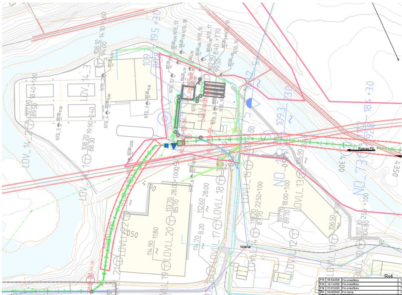
Figur 15 Plantegning med va-trase og aktuelle borpunkt. På enkelte borpunkt mangler symbol for prøvetaking og CPTu'er. For mer detaljer om utførte grunnundersøkelser på tomten vises det til borplan og oversikt i Tabell 1.
