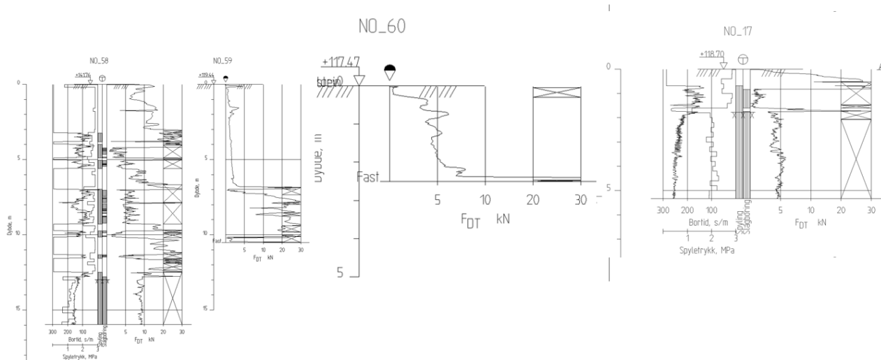
Figur 38 Aktuelle borpunkt utført av Norconsult, NO_059 er tatt i bunn av skråning, NO_058 er tatt i topp, NO_017 og NO_060 er tatt videre bortover flata
