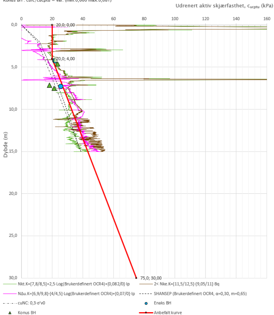
Figur 3 Designprofil for C_u basert på trykksondering og laboratorieundersøkelser i borhull 68.
