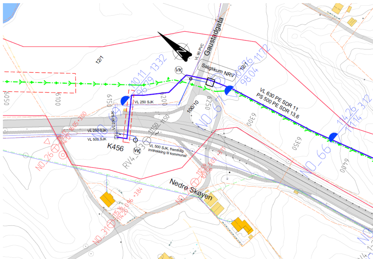
Figur 22 Plantegning med va-trase og aktuelle borpunkt
