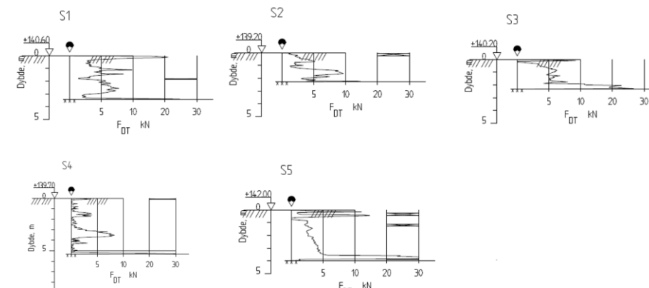
Figur 44 Borpunkt utført av SVV [22]
