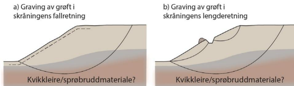
Figur 9 Graving av grøft på inntil to meters dybde i skråning
