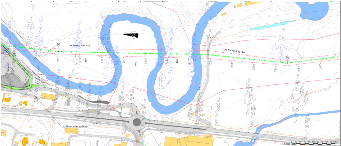
Figur 17 Plantegning med VA-trase og aktuelle borpunkt
