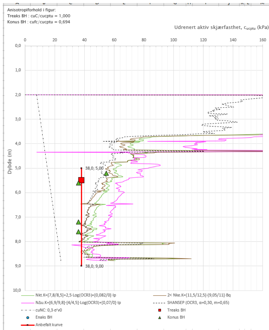
Figur 9 Designprofil for Cu basert på trykksondering og laboratorieundersøkelser i borhull NO_61.
