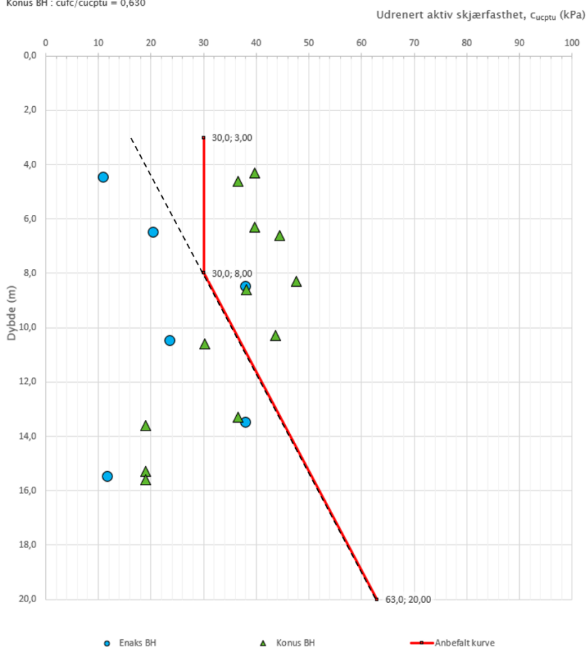
Figur 2 Designprofil for Cu basert på laboratorieundersøkelser i borhull 16230_2. SHANSEP-linjen er illustrert med stiplet linje.
