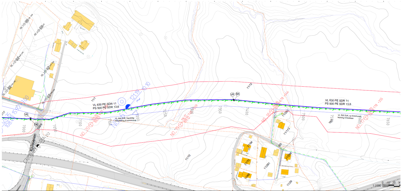
Figur 32 Plantegning va-trase
