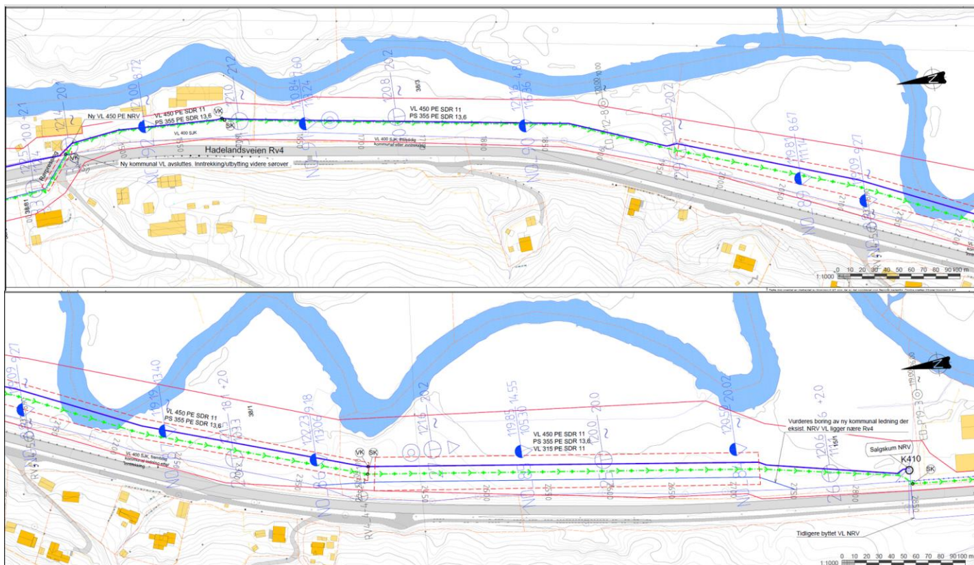
Figur 11 Plantegning med va-trase og aktuelle borpunkt
