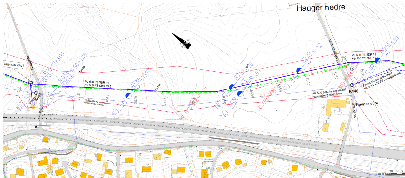
Figur 39 Plantegning med VA-trase og aktuelle borpunkt
