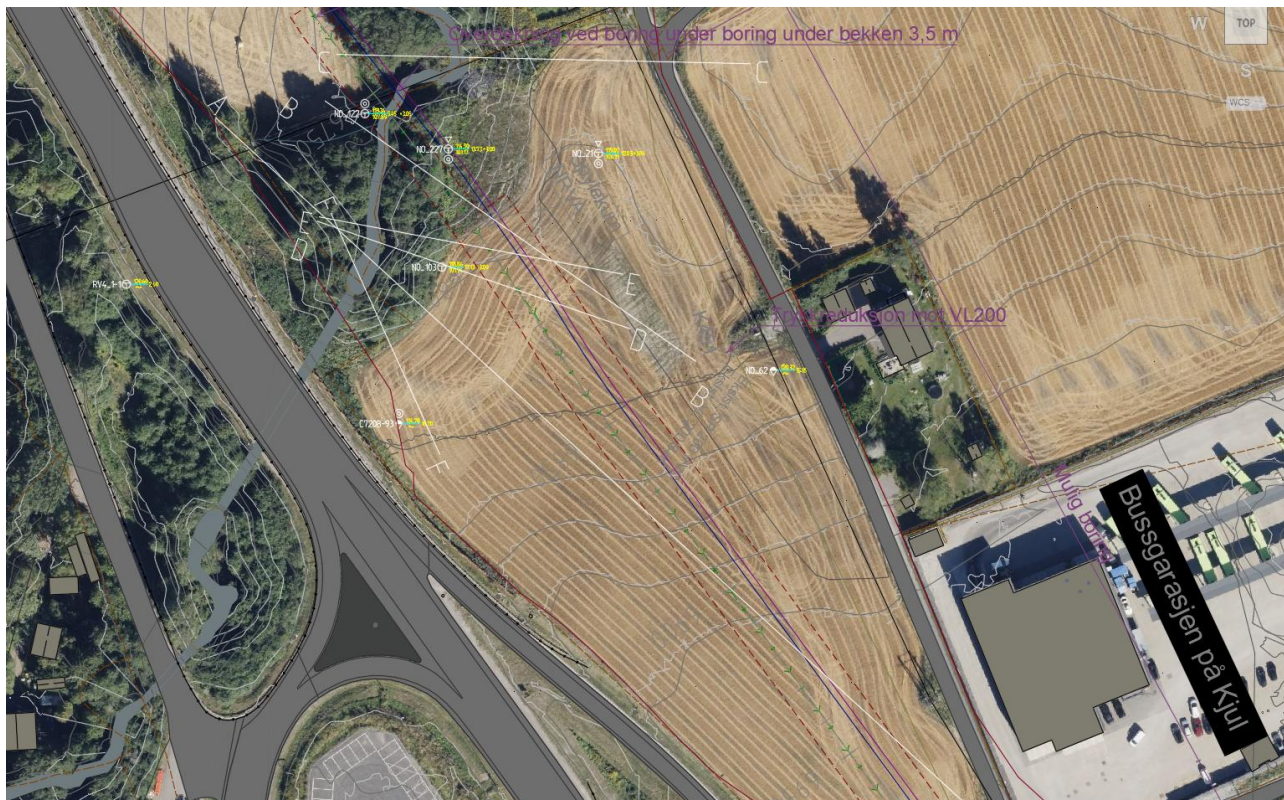
Figur 65 Plassering av snitt A-F i sone Kjøl.
