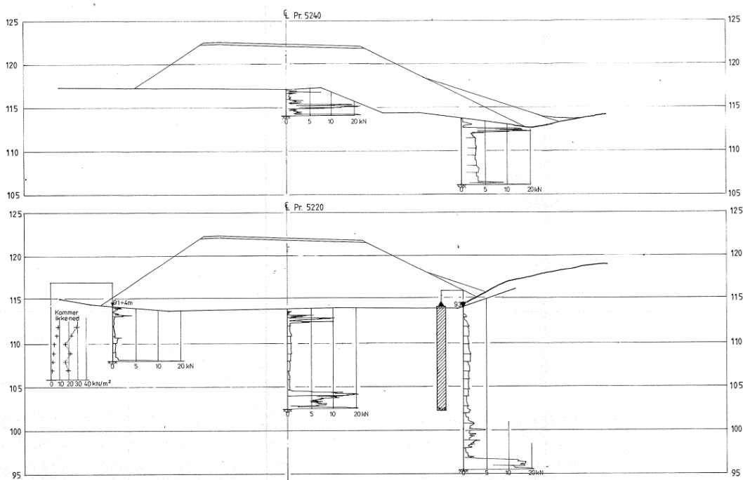
Figur 69 Skissert fylling for Rv. 4, samt motfylling ved bekken til kote +116.
