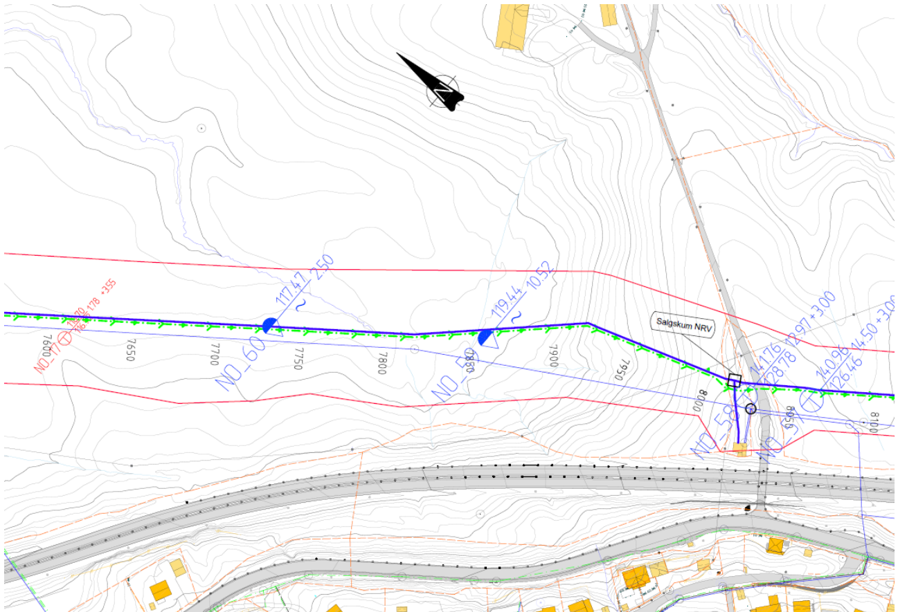
Figur 36 Plantegning med va-trase og aktuelle borpunkt
