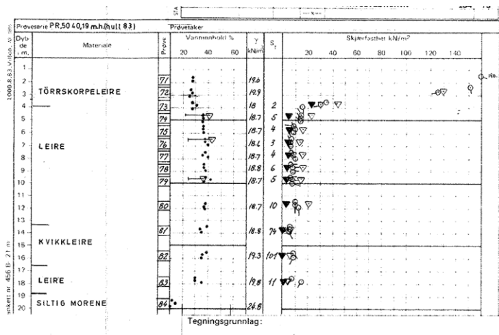
Figur 34: Utklipp fra prøveanalyse i posisjon C720B-83. Denne viser kvikkleire i dybdesjiktet 13-16,5 m (tilsvarer kt +111,6 til +108,1), [13]
