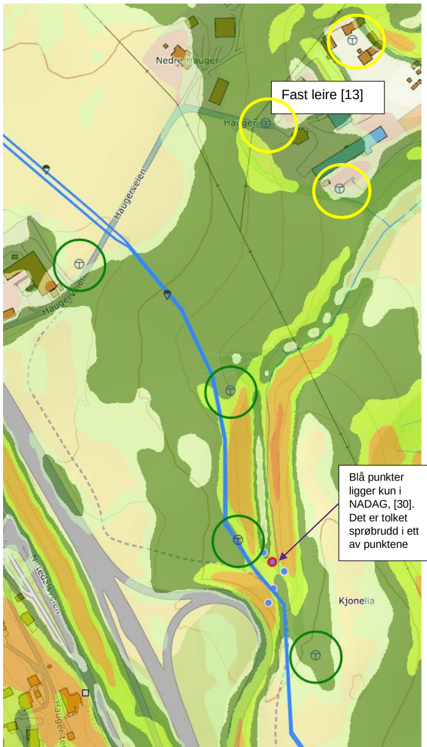
Figur 45 Oversiktsbilde med terrenghelning, borpunkt med tolket kvikkleire og skissert va-trase. Gul sirkel indikerer leire, oransje sirkel er antatt sprøbrudd og rød er påvist sprøbrudd. Grønn er enten påvist ikke sprøbrudd eller tolket å ikke inneholde leire.
