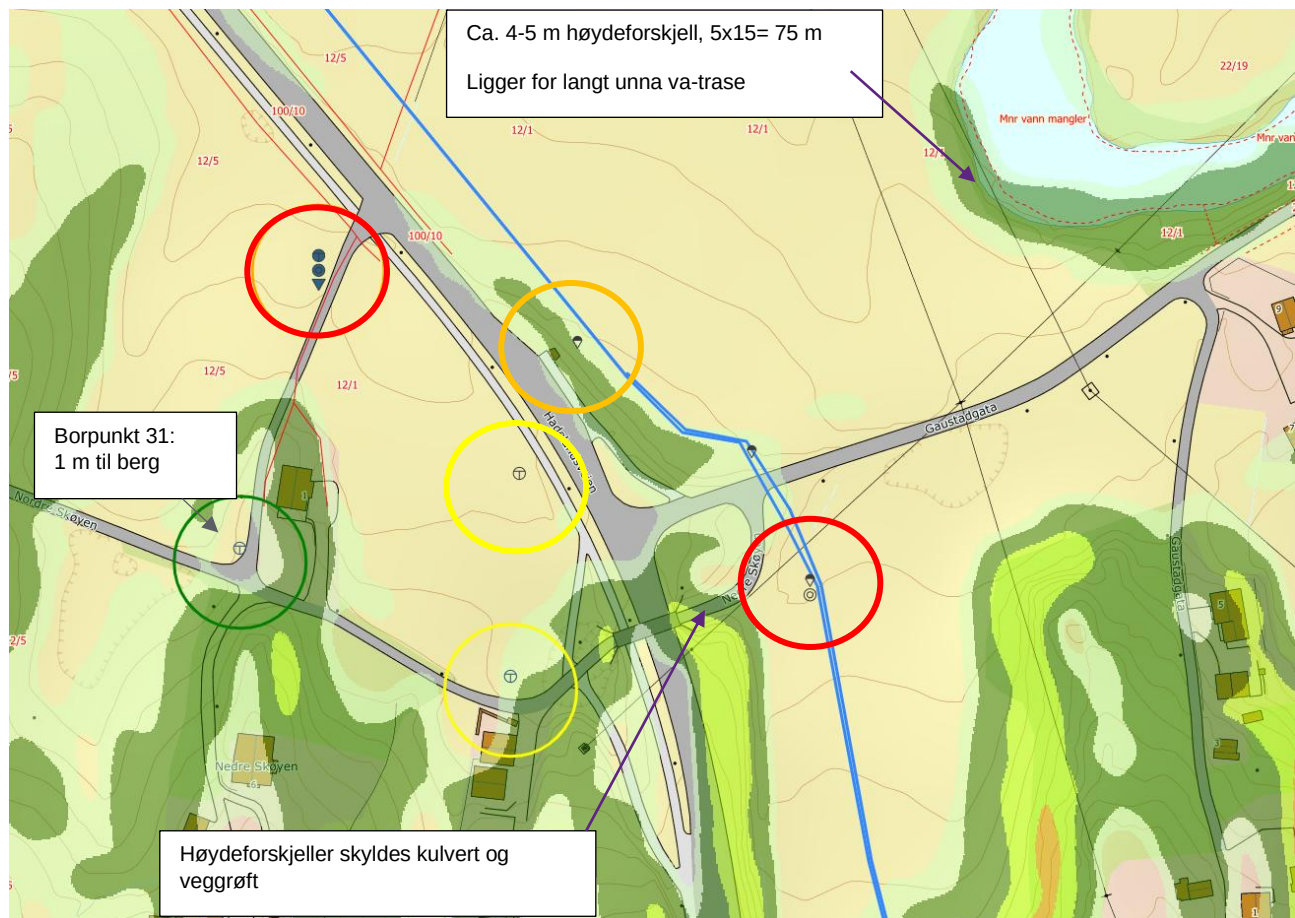
Figur 23 Oversiktsbilde med terrenghelning, borpunkt med tolket kvikkleire og skissert va-trase. Gul sirkel indikerer leire, oransje sirkel er antatt sprøbrudd og rød er påvist sprøbrudd. Grønn er enten påvist ikke sprøbrudd eller tolket å ikke inneholde leire.
