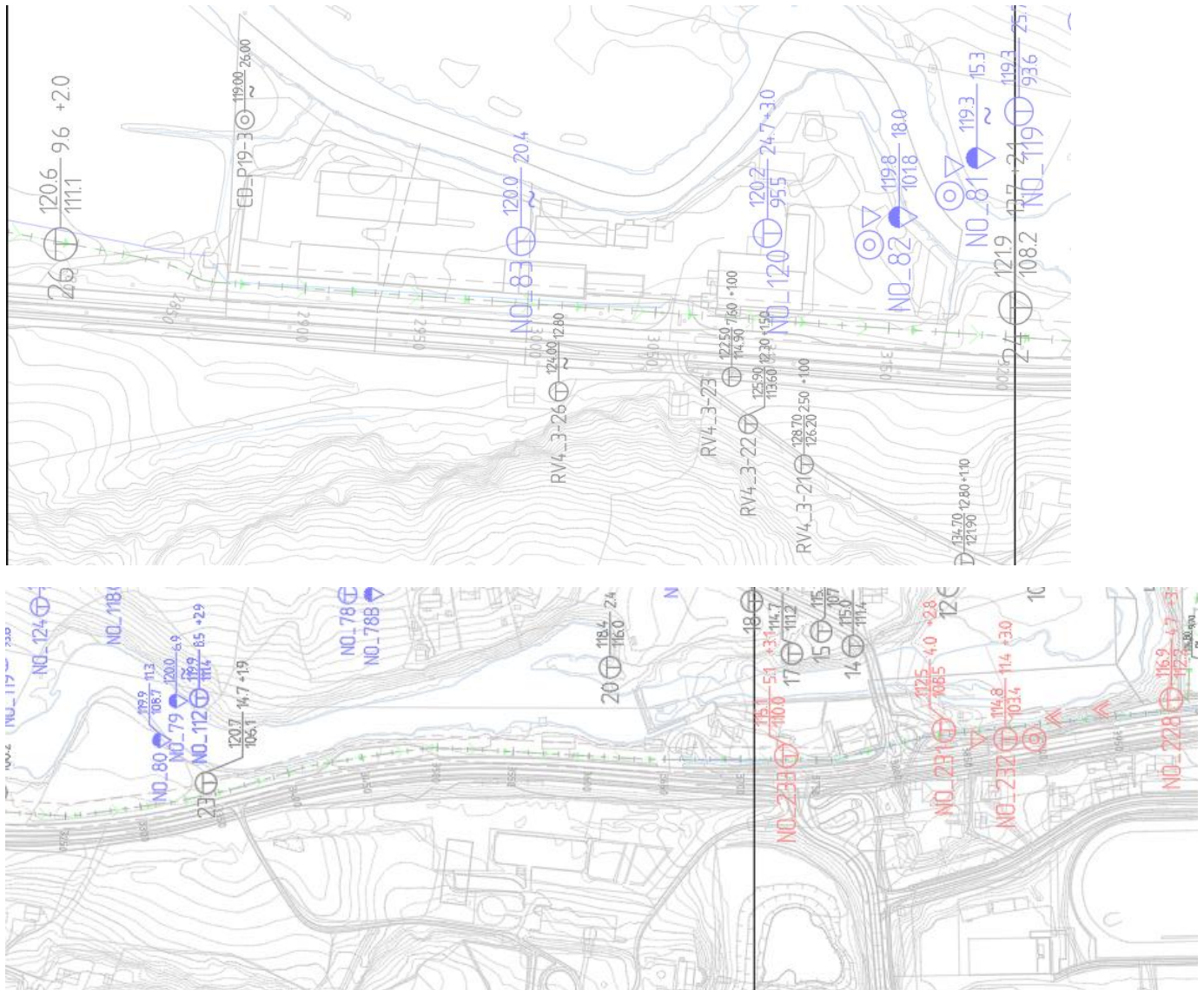
Figur 13 Plantegning med va-trase og borpunkt
