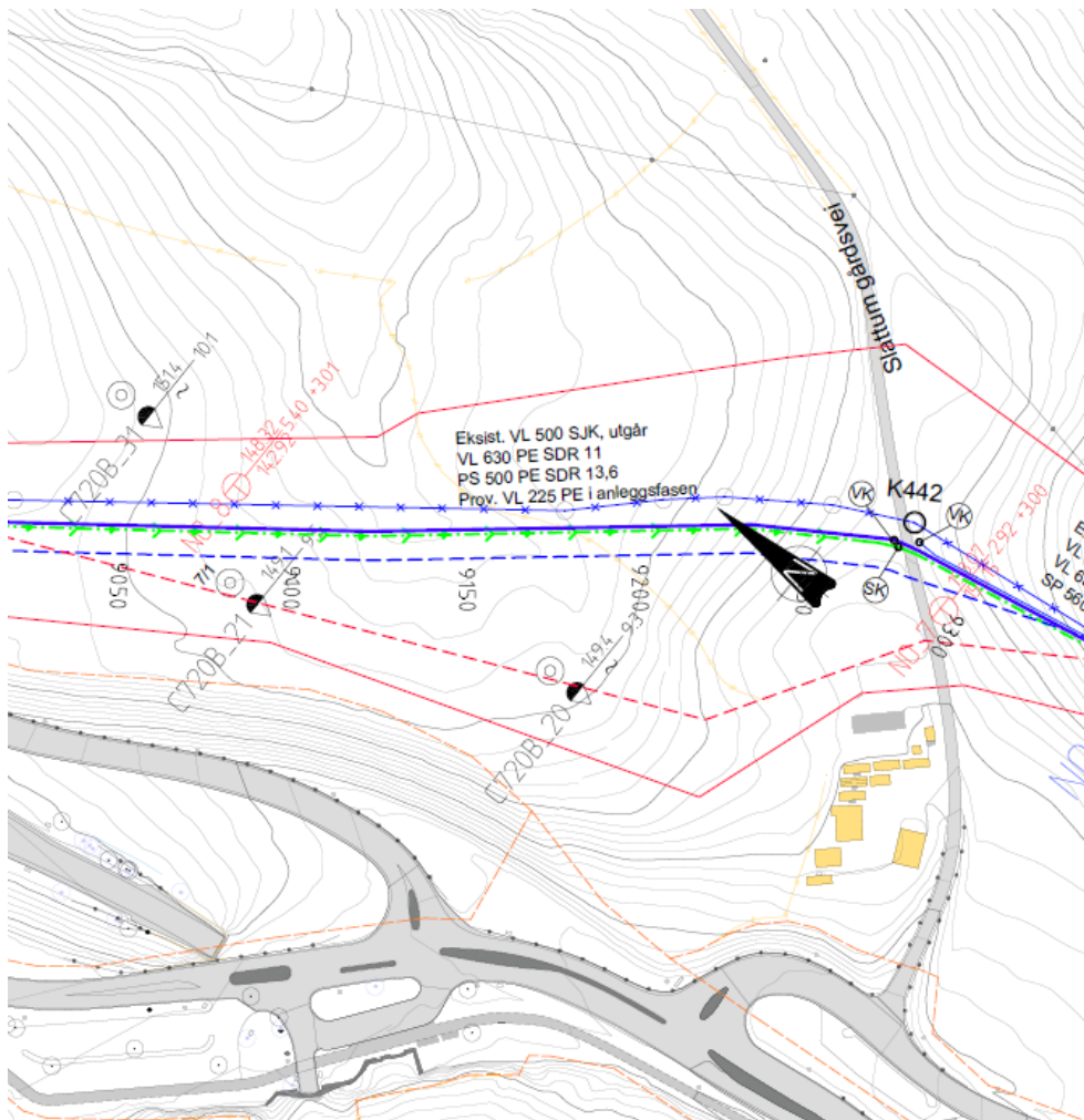
Figur 47 Plantegning med va-trase og aktuelle borpunkt
