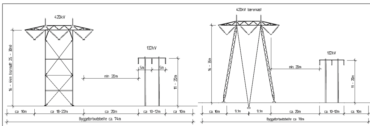
Figur 12: Skisse av master for ny 420 kV ledning ved parallelføring med eksisterende 132 kV ledning. Til venstre ved bruk av selv bærende mast, og til høyre med utvendig bardunert mast. Bredden på ryddegaten og byggeforbudsbeltet blir da rett i overkant av 70 m.
