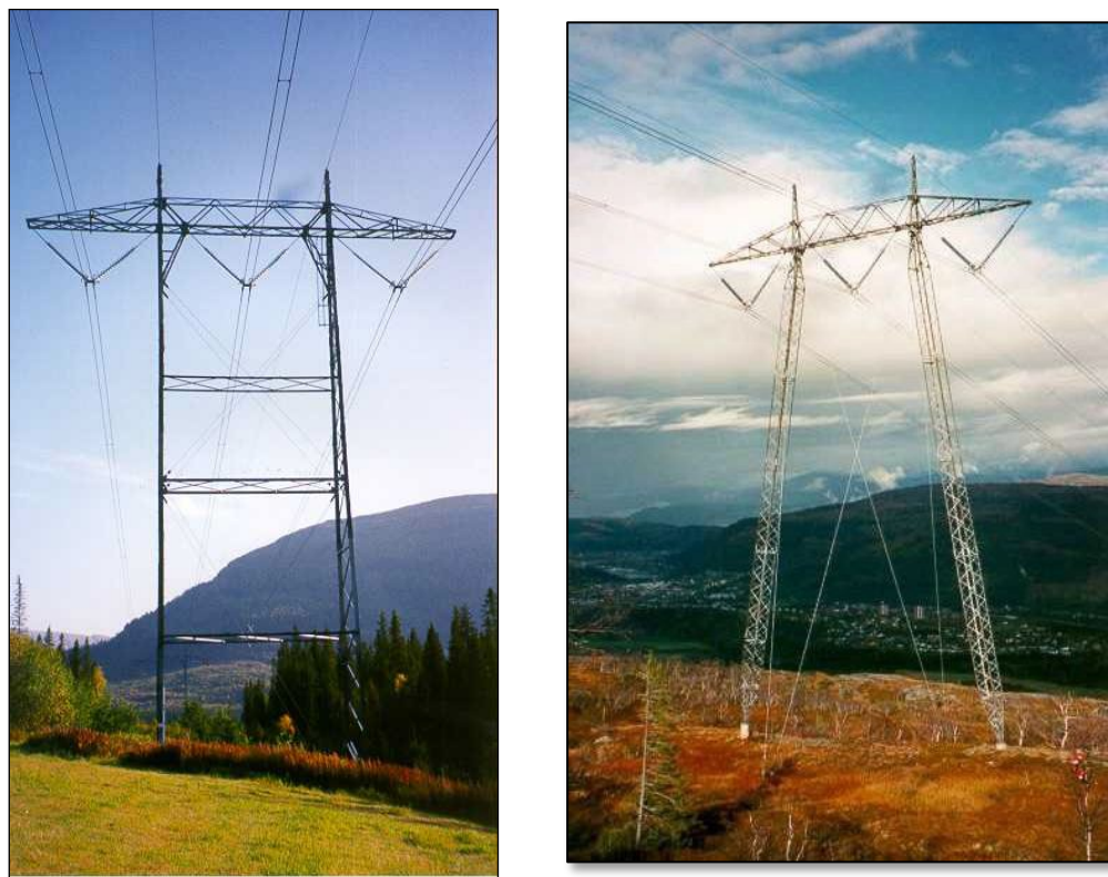
Figur 11: Bilder av aktuelle mastetyper for 420 kV ledning, til venstre selv bærende stålmast, til høyre utvendig bardunert mast (M-mast).
