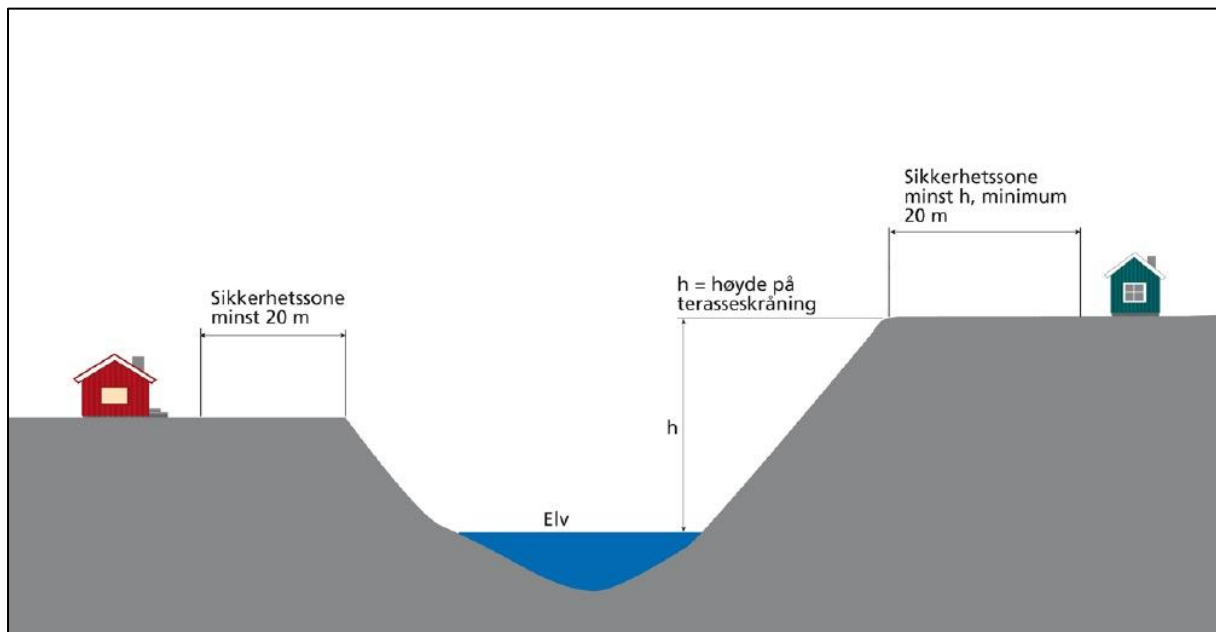
Figur 14: Illustrasjon av sikkerhetssone mot erosjon (gjengitt fra TEK17 §7-2 fjerde ledd).
