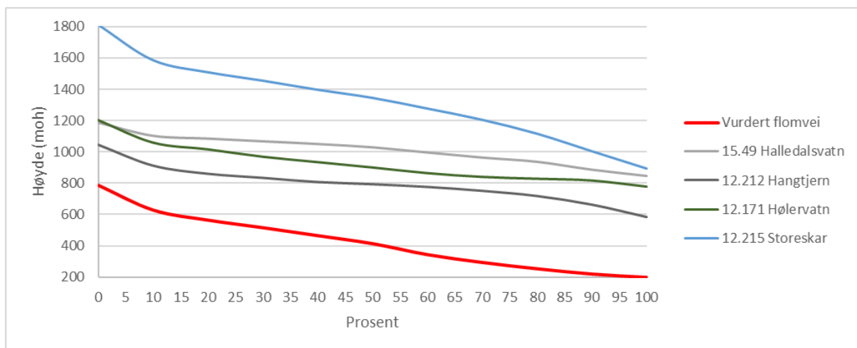
Figur 7: Høydefordelinga til flomveien og vurderte målestasjoner.
