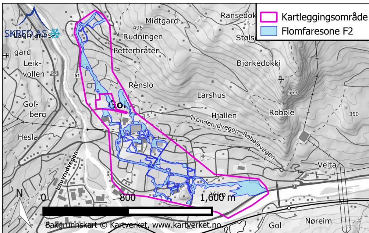
Figur 15: Faresone for 200-årsflom med klimapåslag (sikkerhetsklasse F2 i TEK17).
