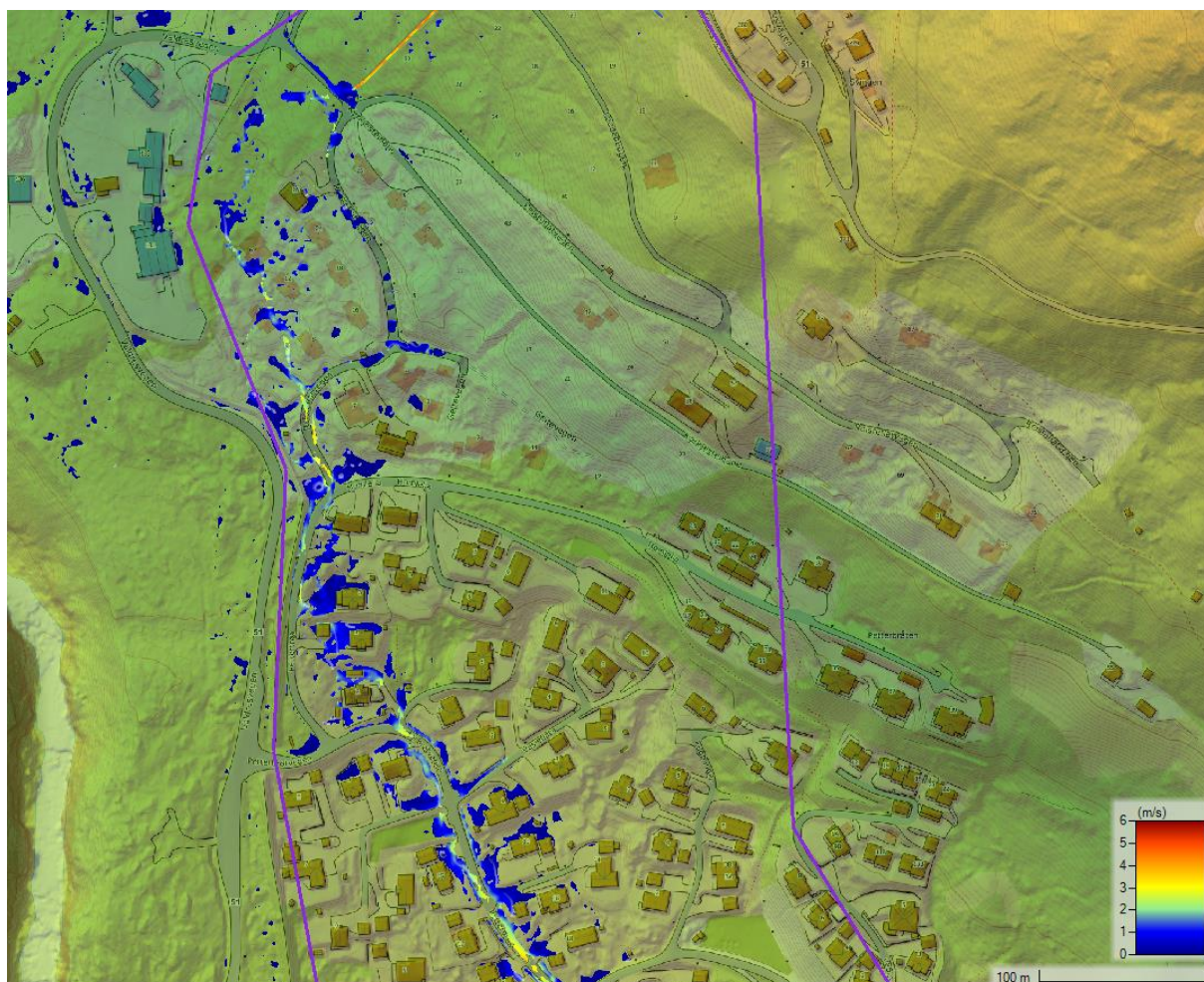
Figur 11: Illustrasjon av modellert strømmingssituasjon i øvre del av kartleggingsområdet ved en 200-årsflom inkludert klimapåslag. Vanndybder større enn 5 cm er vist.
