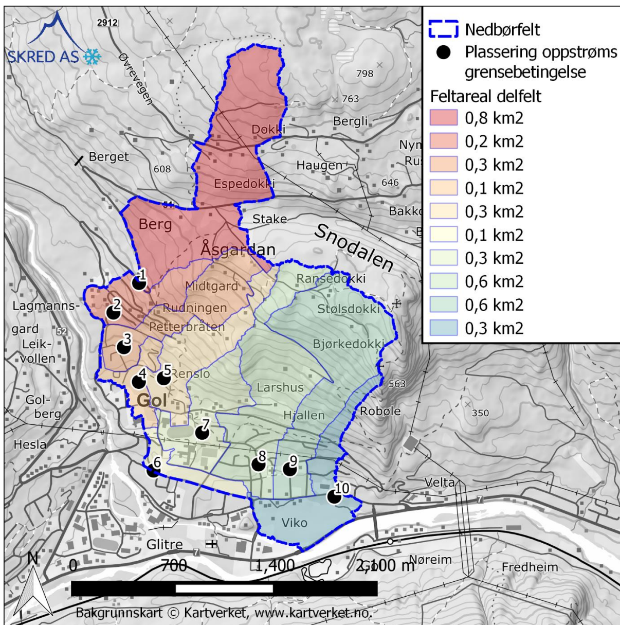
Figur 8: Inndeling av nedbørfeltet i delfelt for fordeling utover i den hydrauliske modellen.
