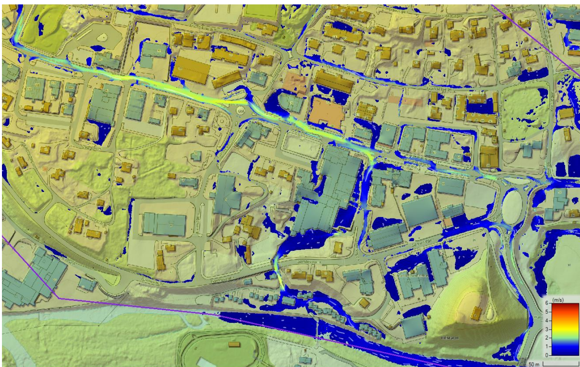
Figur 13: Illustrasjon av modellert strømningssituasjon langs Sentrumsvegne og nedre del ved en 200-årsflom inkludert klimapåslag. Vanddybder større enn 5 cm er vist.
