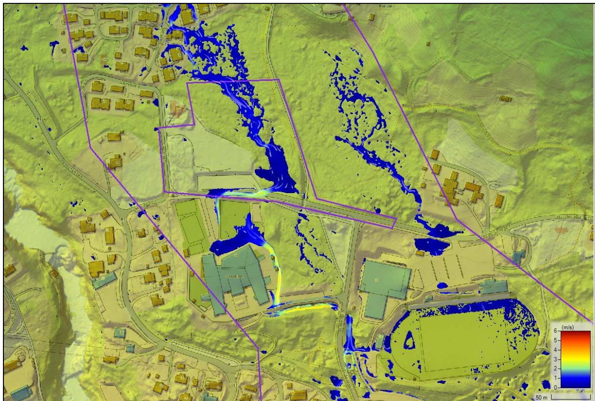
Figur 12: Illustrasjon av modellert strømningssituasjon forbi barnehagetomta (i lilla) ved en 200-årsflom inkludert klimapåslag. Vanddybder større enn 5 cm er vist.
