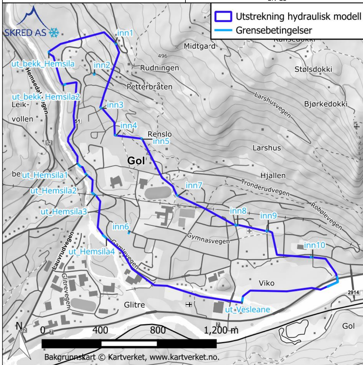
Figur 9: Utstrekning til hydraulisk modell.
