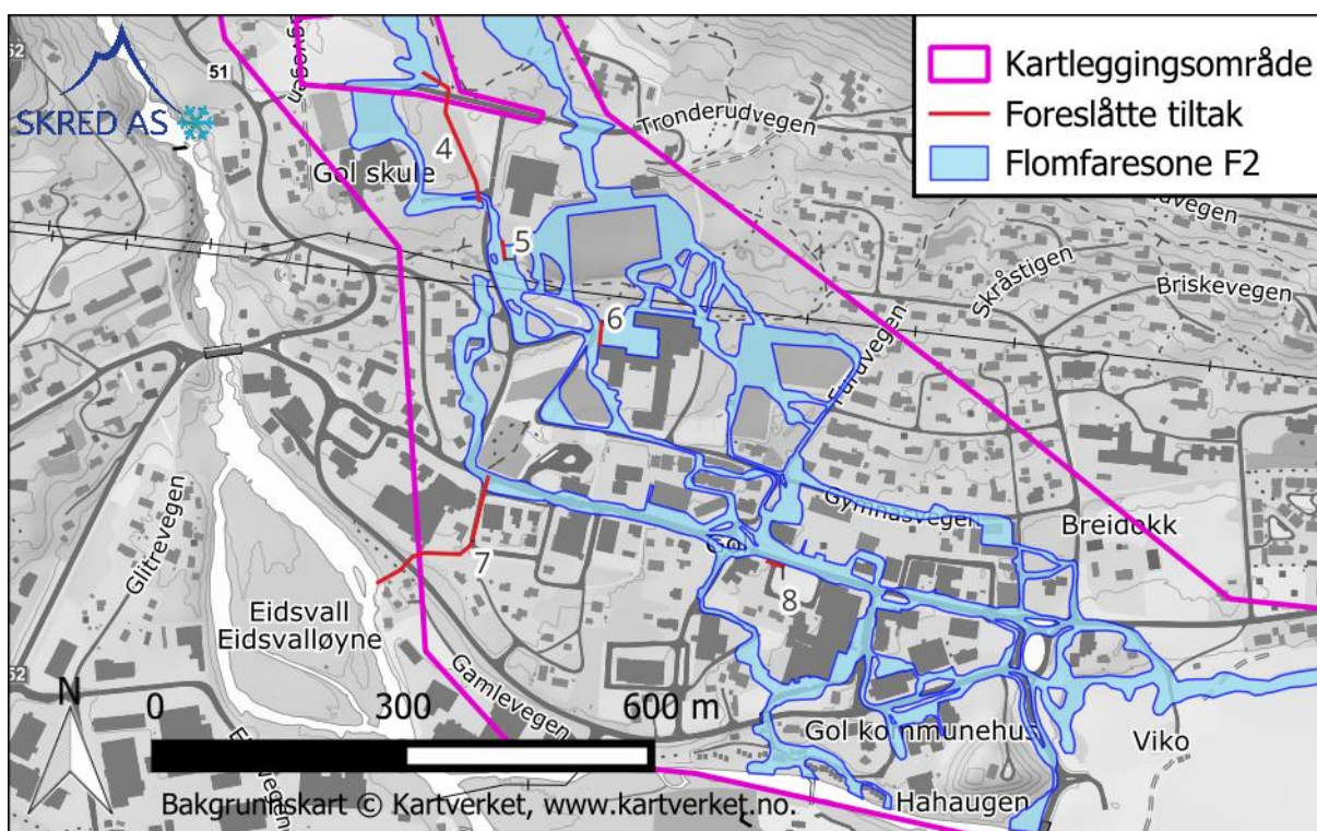
Figur 17: Foreslåtte tiltak og faresoner i nedre del av kartleggingsområdet.
