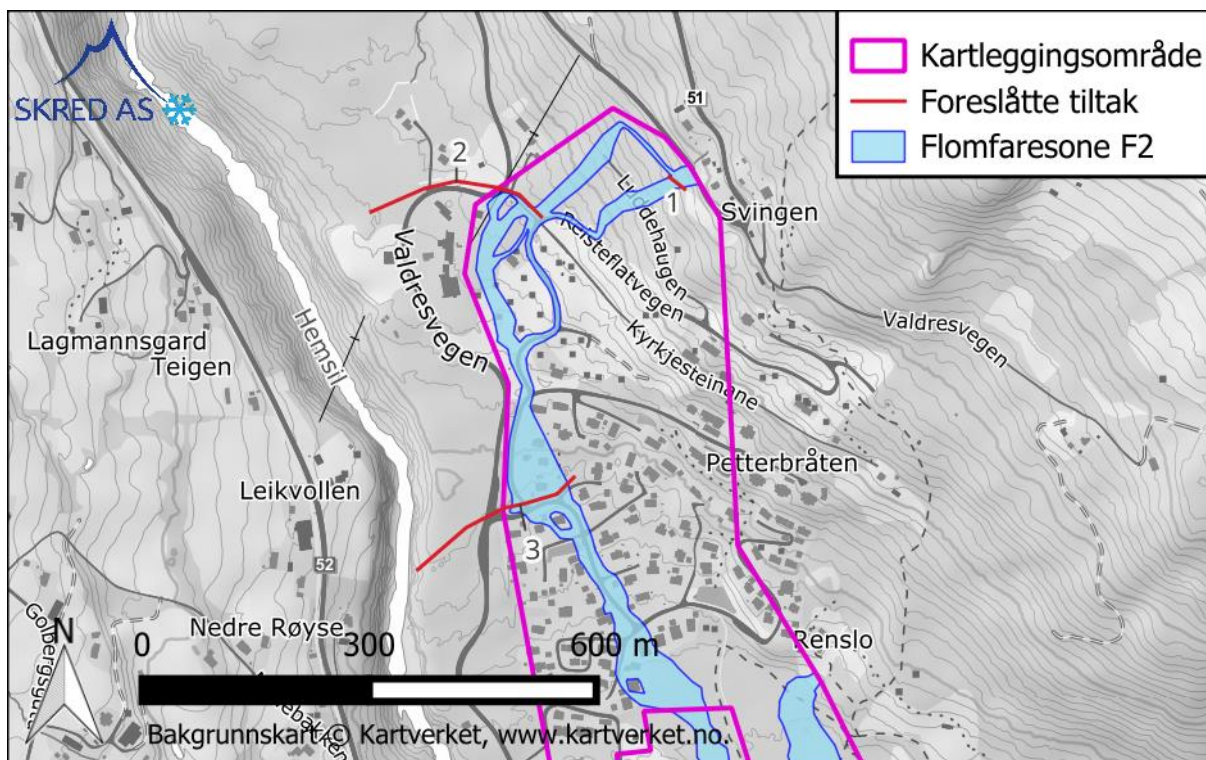
Figur 16: Foreslåtte tiltak og faresoner i øvre del av kartleggingsområdet.
