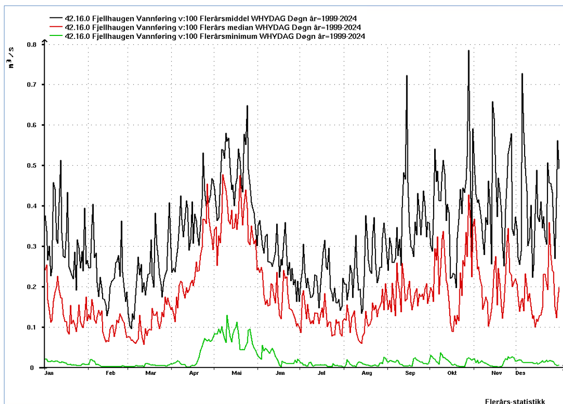
Fig. 5: Sesongvariasjonene i m^3/s i Haugåna, basert på flerårs døgnaverdier.
