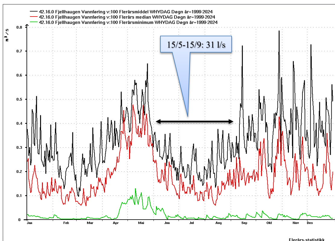
Fig.17: Minstevannføringen maksimeres i den viktigste vekstperioden
