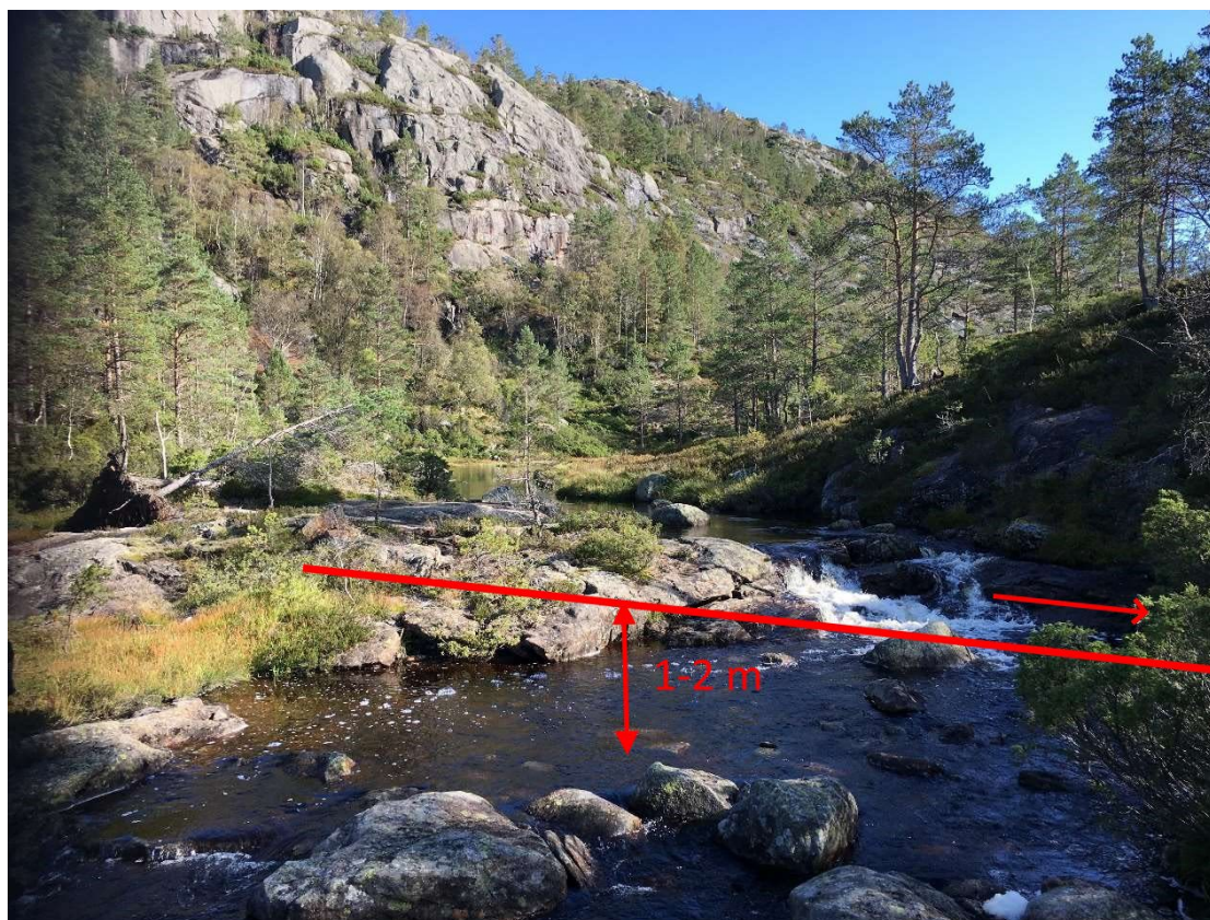
Fig. 8: Planlagt område for hovedinntak m/inntaksterskel i forgrunnen. Vannet ledes mot inntakskum i høyre billedkant (Foto: Småkraftkonsult)
