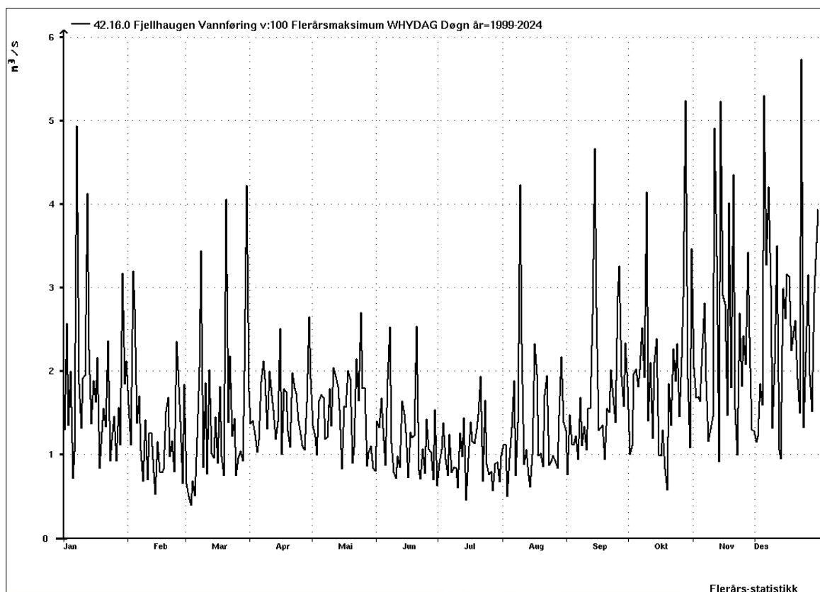
Fig. 6: Maksimale flommer som døgnmiddel m^3/s i Haugåna
