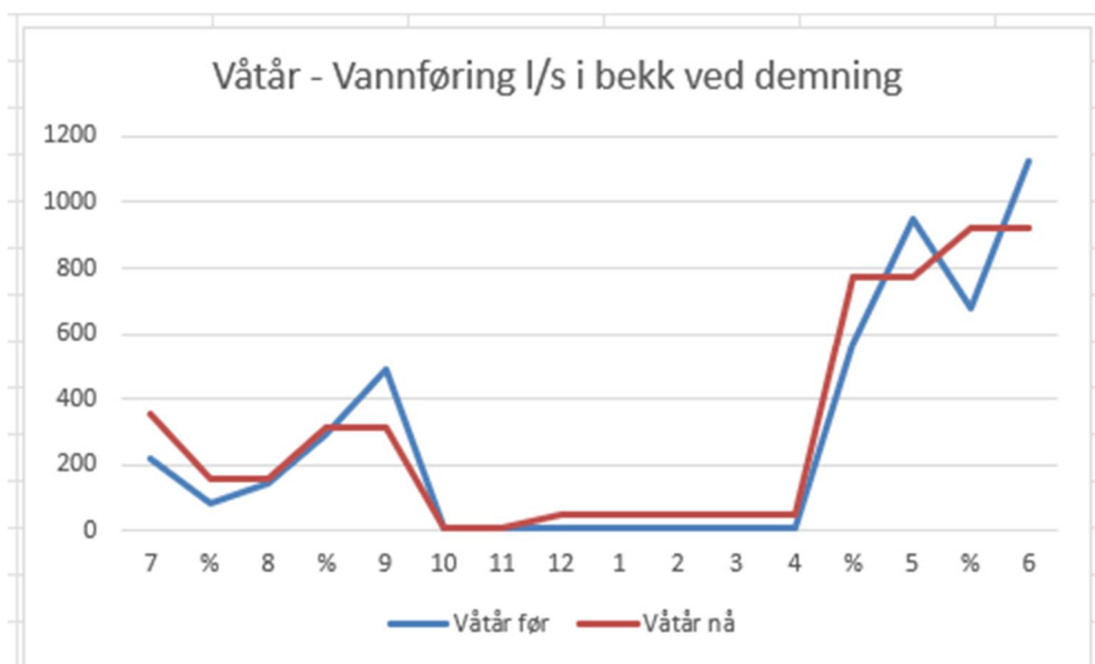
Fig. 3.1d Vannføring Våtår (1976 Sandåmo Namsskogan)
