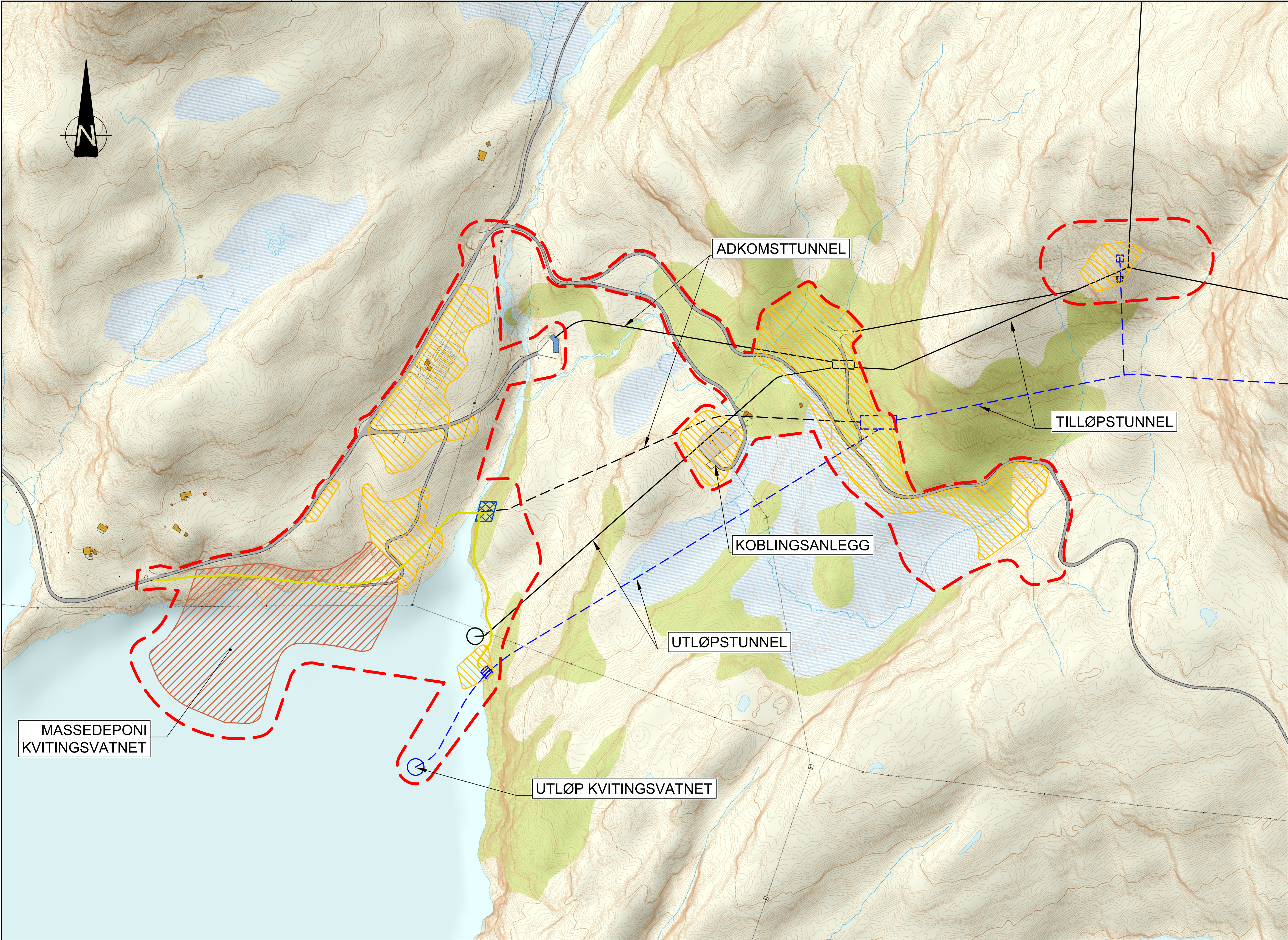
OVERSIKT KVITINGSVATNET 1:2 500
