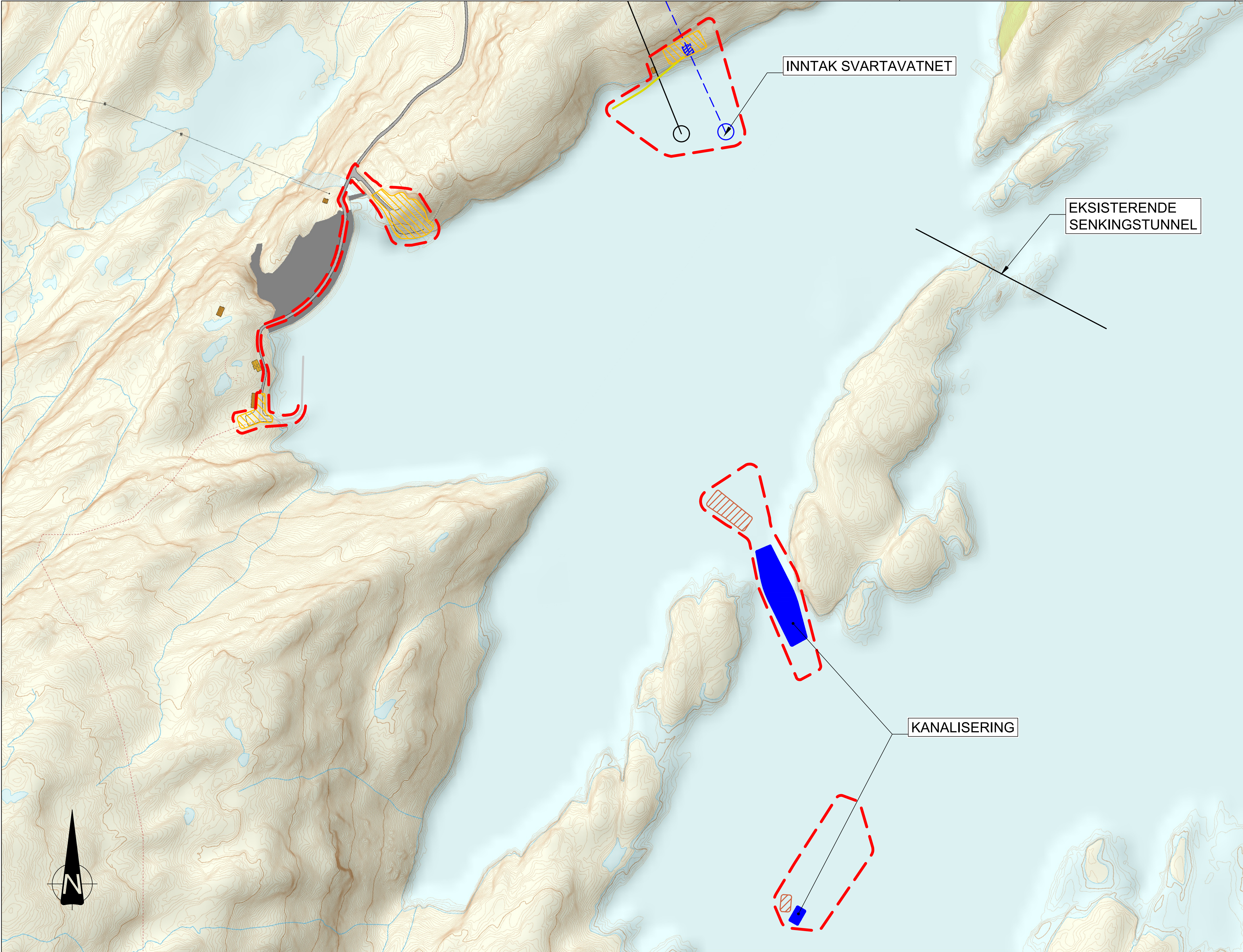
OVERSIKT SVARTAVATNET 1:2 500
