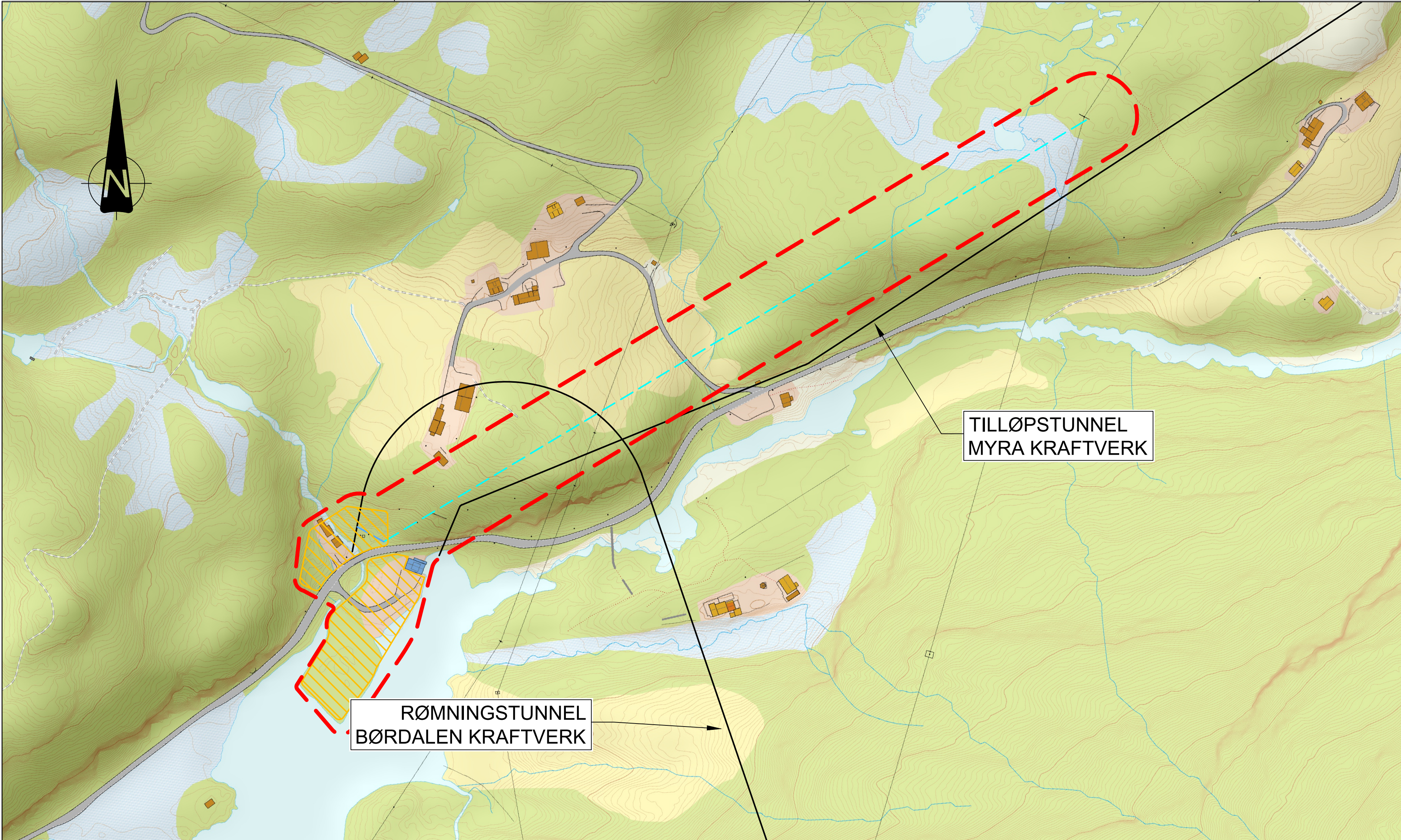
OVERSIKT MYRA 1:2 000
