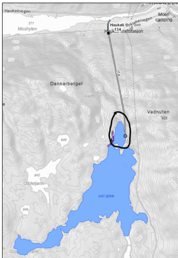
Figur 1: Skartjern (sort sirkel) omfatter nedre del av Vatjern som er inntaksbassenget til Haukeli Kraftverk.
