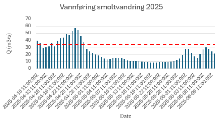
Figur 1. Vannføring ved Boenfoss (målestasjon Flakksvann) i smoltutvandningsperioden 2025. Ny slukeevne som omfattes av den midlertidige tillatelsen er markert med rødstiplot linje (33 m 3 /s).
