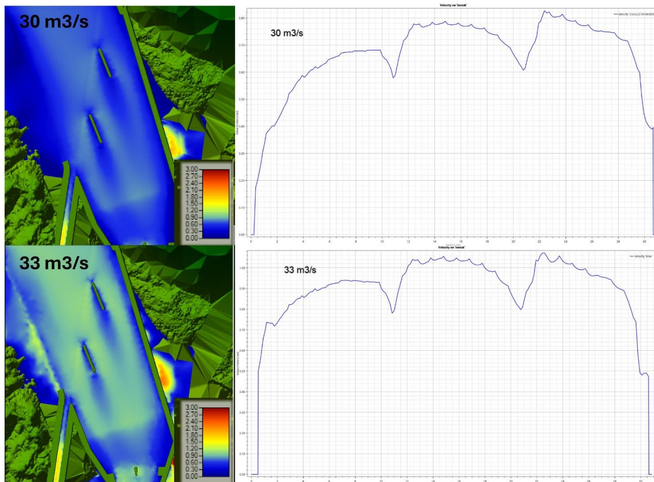
Figur 2-1. Beregnet strømningsmønster og strømningshastighet i strømningsretning, ved vannføring 30 og 33 m³/s. Beregningene viser uniform hastighetsfordeling ved begge de simulerte vannføringene.
