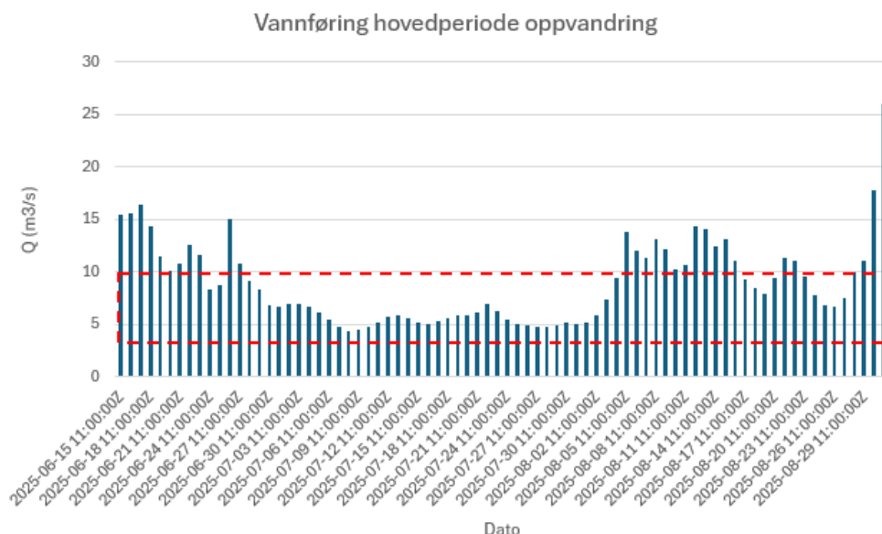
Figur 2. Vannføring ved Boenfoss (målestasjon Flakksvann) i hovedperioden for oppvandring av laks og sjørøret i 2025. Intervall for minstevannføring i undersøkelsesperioden er vist med rødstiplot rektangel (3-10 m³/s).
