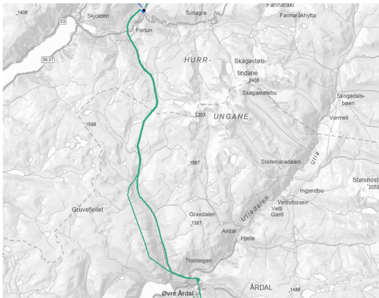
Kart 1: 132 kV-ledningene mellom Jamnane og Øvre Årdal
