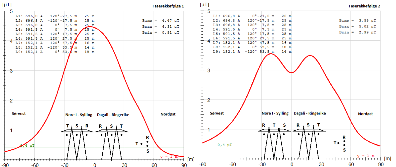
Figur 4 Grafisk fremstilling av magnetfelt rundt de to eksisterende 420 kV luftledningene og den omsøkte 132 kV luftledningen med 132 kV luftledning på nordøstlig side.
