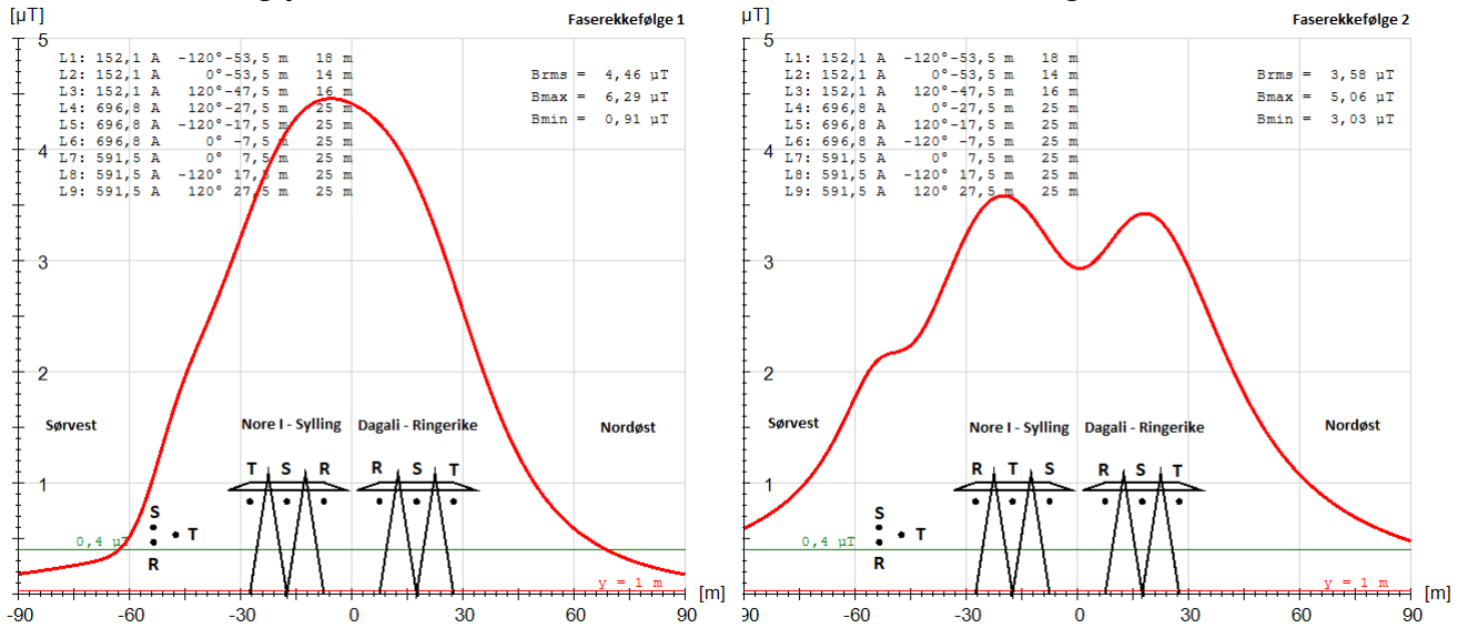
Figur 3 Grafisk fremstilling av magnetfelt rundt de to eksisterende 420 kV luftledningene og den omsøkte 132 kV luftledningen med 132 kV luftledning på sørvestlig side.
