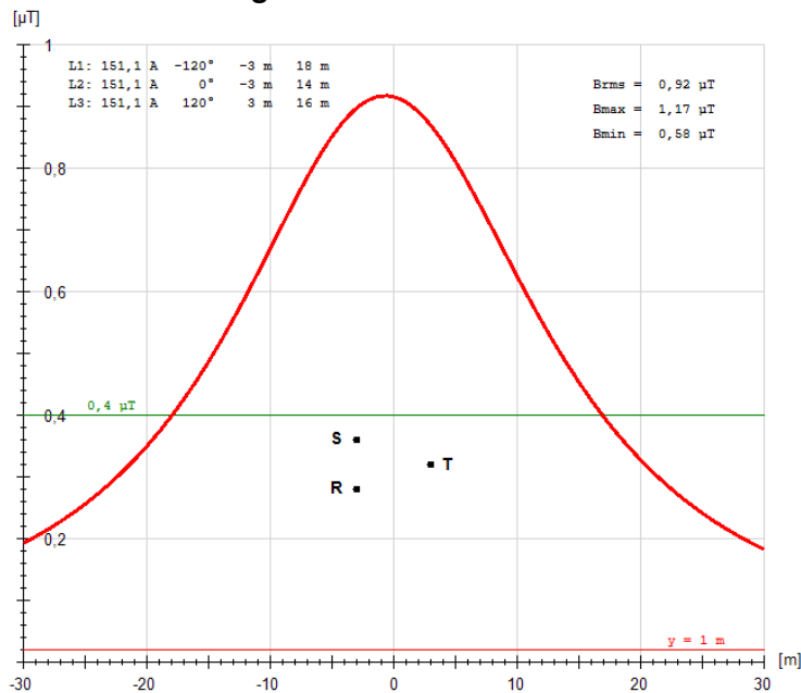
Figur 2 Grafisk fremstilling av magnetfelt rundt den omsøkte 132 kV luftledningen.
