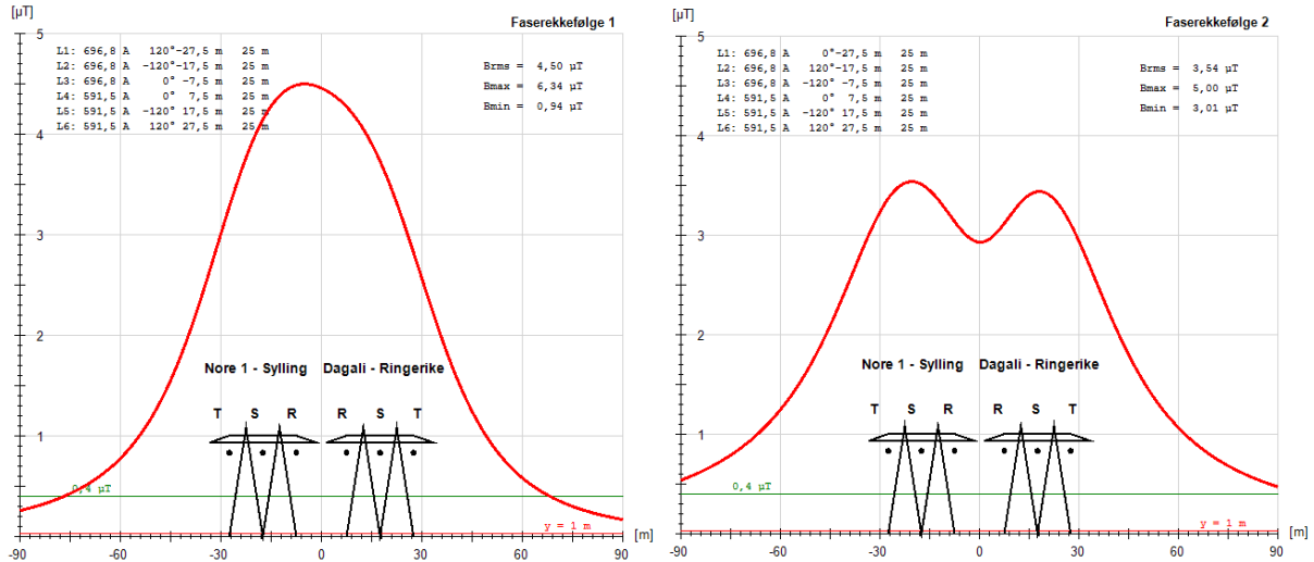
Figur 1 Grafisk fremstilling av magnetfelt rundt de to eksisterende 420 kV luftledningene.
