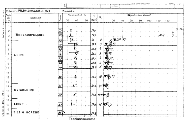
Figur 34: Utklipp fra prøveanalyse i posisjon C720B-83. Denne viser kvikkleire i dybdesjiktet 13-16,5 m (tilsvarer kt +111,6 til +108,1), [13]
