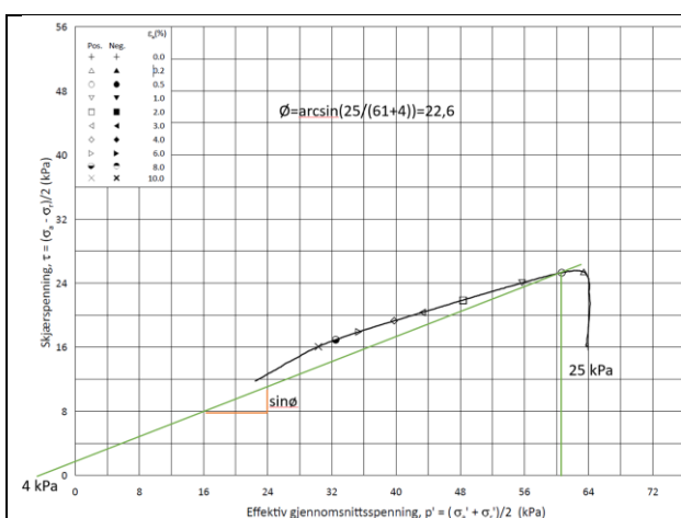
Figur 4 Tolket friksjonsvinkel og attraksjon fra treaksforsøk i NO_21. Forsøket har lav kvalitet.
