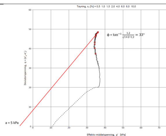
Figur 5 Tolket friksjonsvinkel og attraksjon fra treaksforsøk i NO_227. Forsøket har høy kvalitet.
