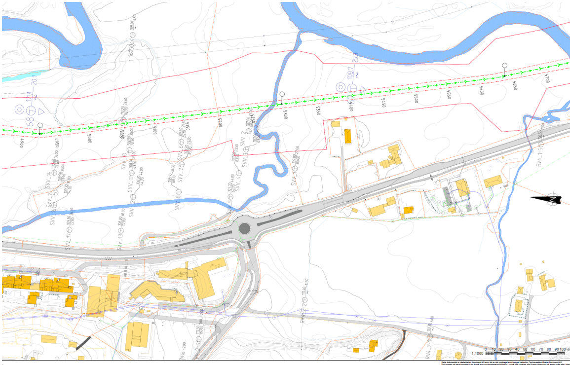
Figur 19 Plantegning med va-trase og aktuelle borpunkt
