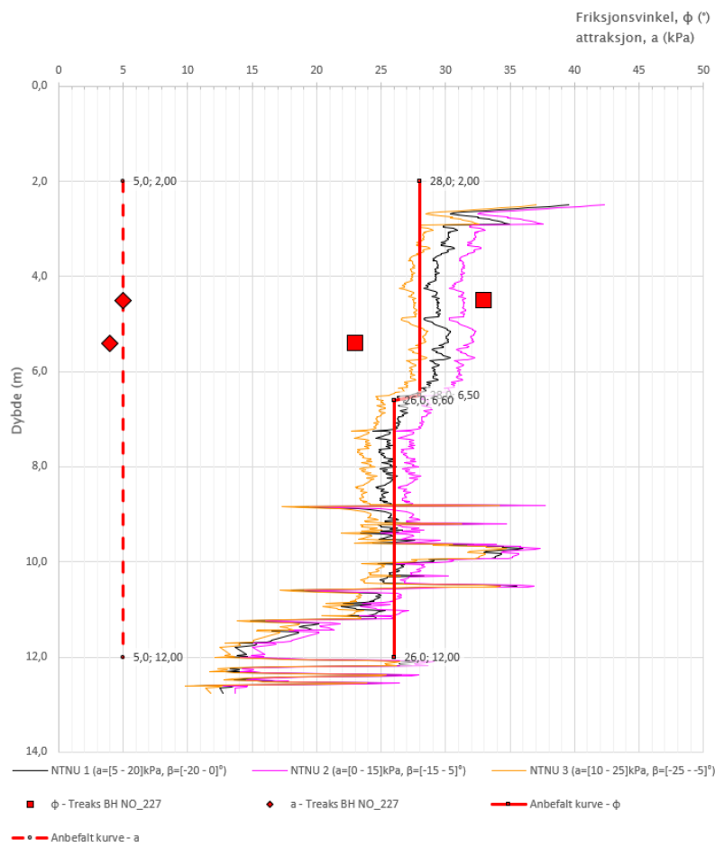
Figur 6 Attraksjon og friksjonsvinkel basert på CPTU og treksforsøk i NO_227 og NO_21. Det er konservativt benyttet friksjonsvinkel 26^\circ i hele leirelaget.
