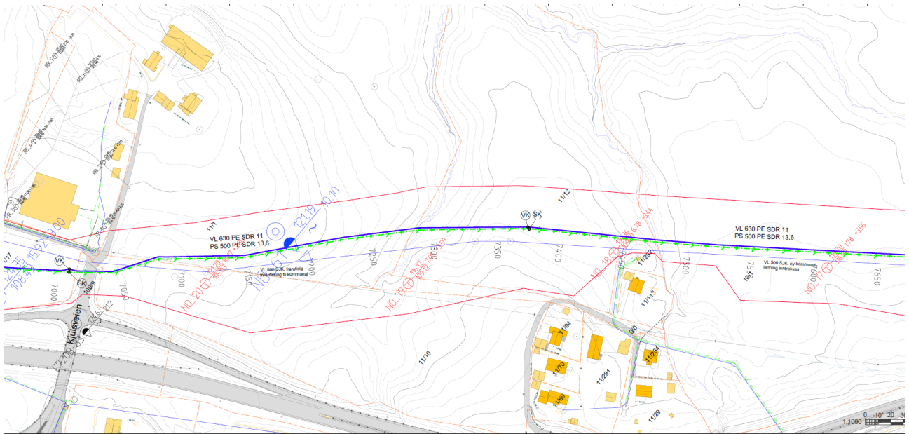
Figur 32 Plantegning va-trase
