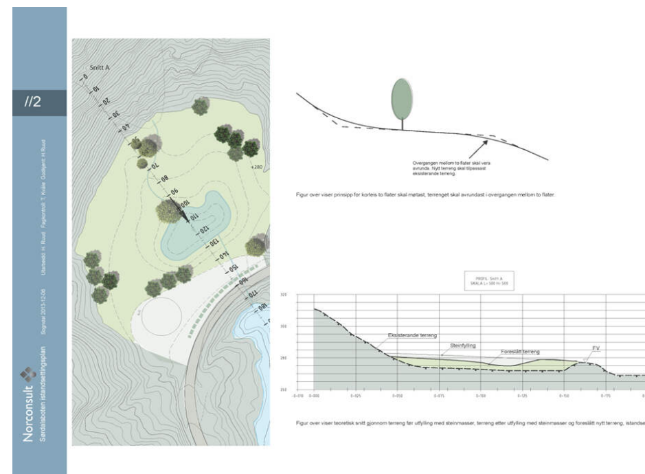
Figur 45: Eksempel på plan for større massedeponi. Planen viser utstrekning, profil og prinsipp for overgang mellom opprinnelig terreng og deponi.
