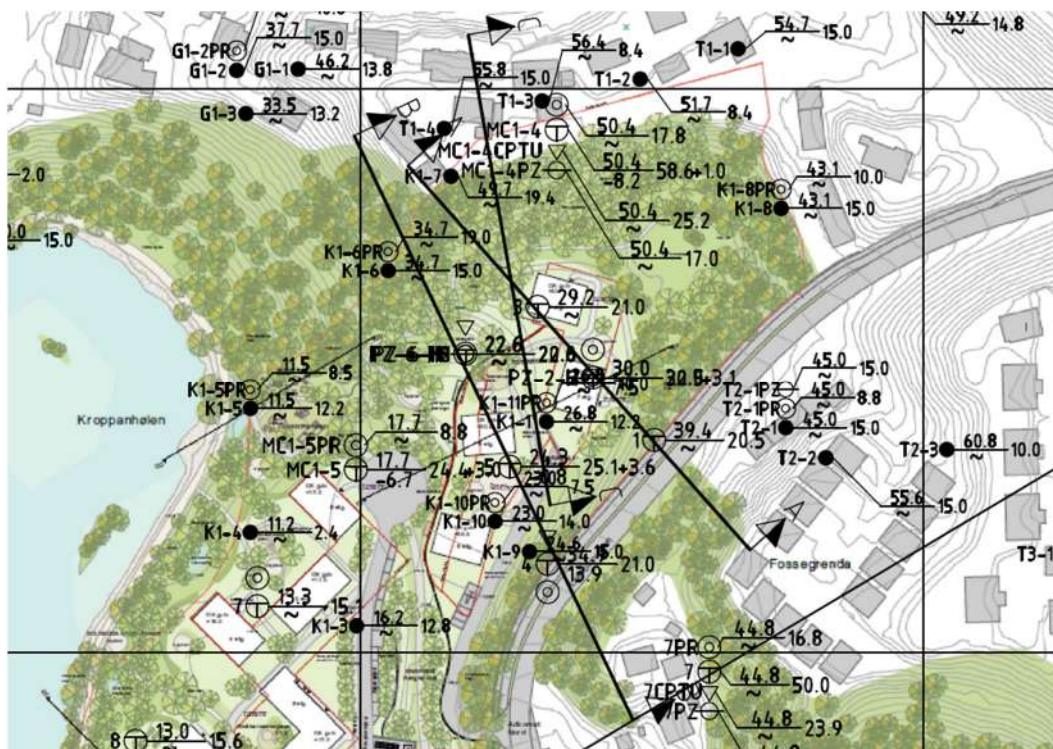
Figur 8-1 Plassering av profiler for stabilitetsberegninger mht. planlagt bebyggelse i ravedalen som vises i /40/ Resultater fra stabilitetsberegninger er vist i tegninger nr. 10247156-RIG-TEG-800.1 t.o.m. 803.2.
